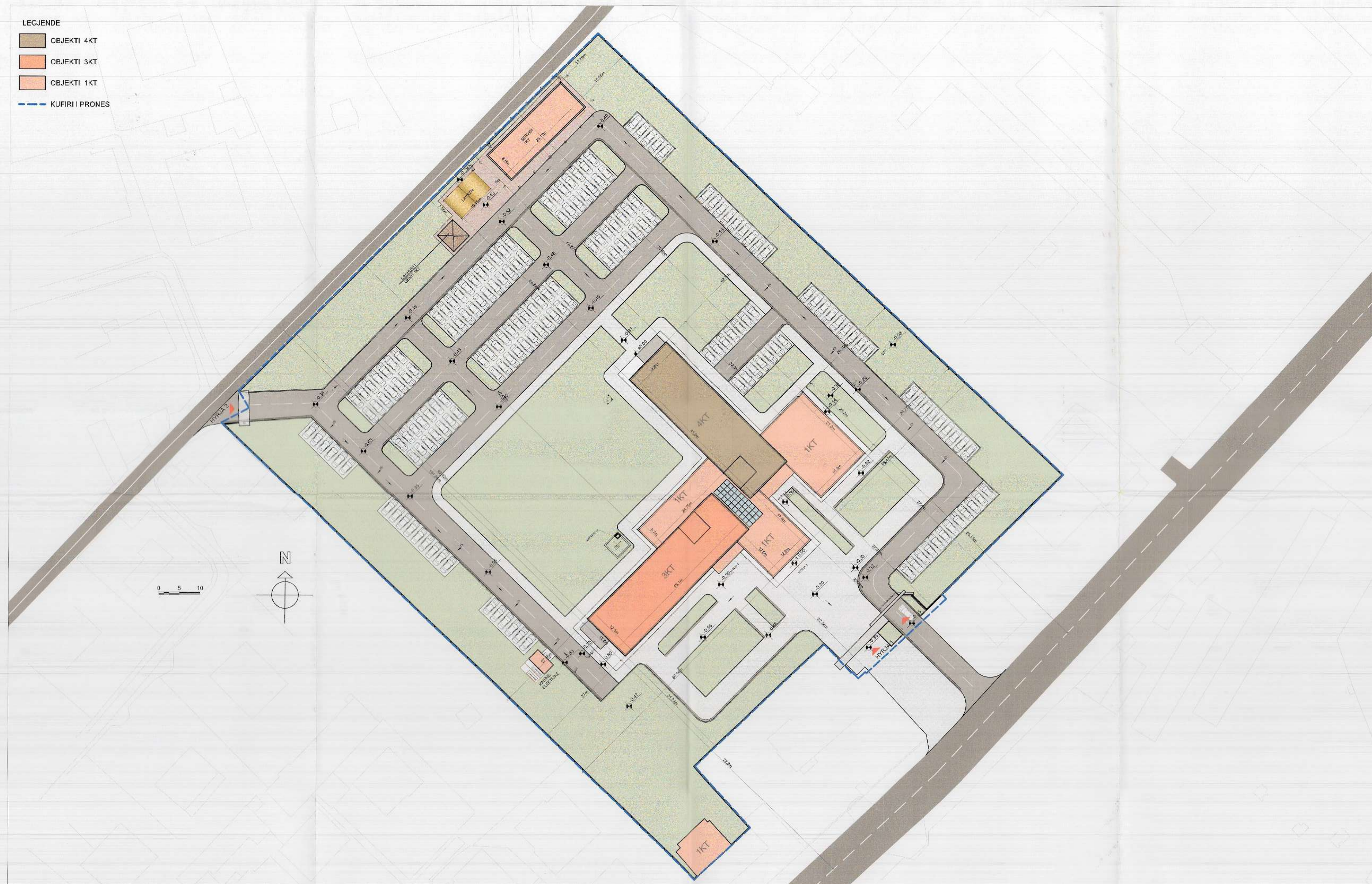
PLANI I VENDOSJES SHK. 1: 500
