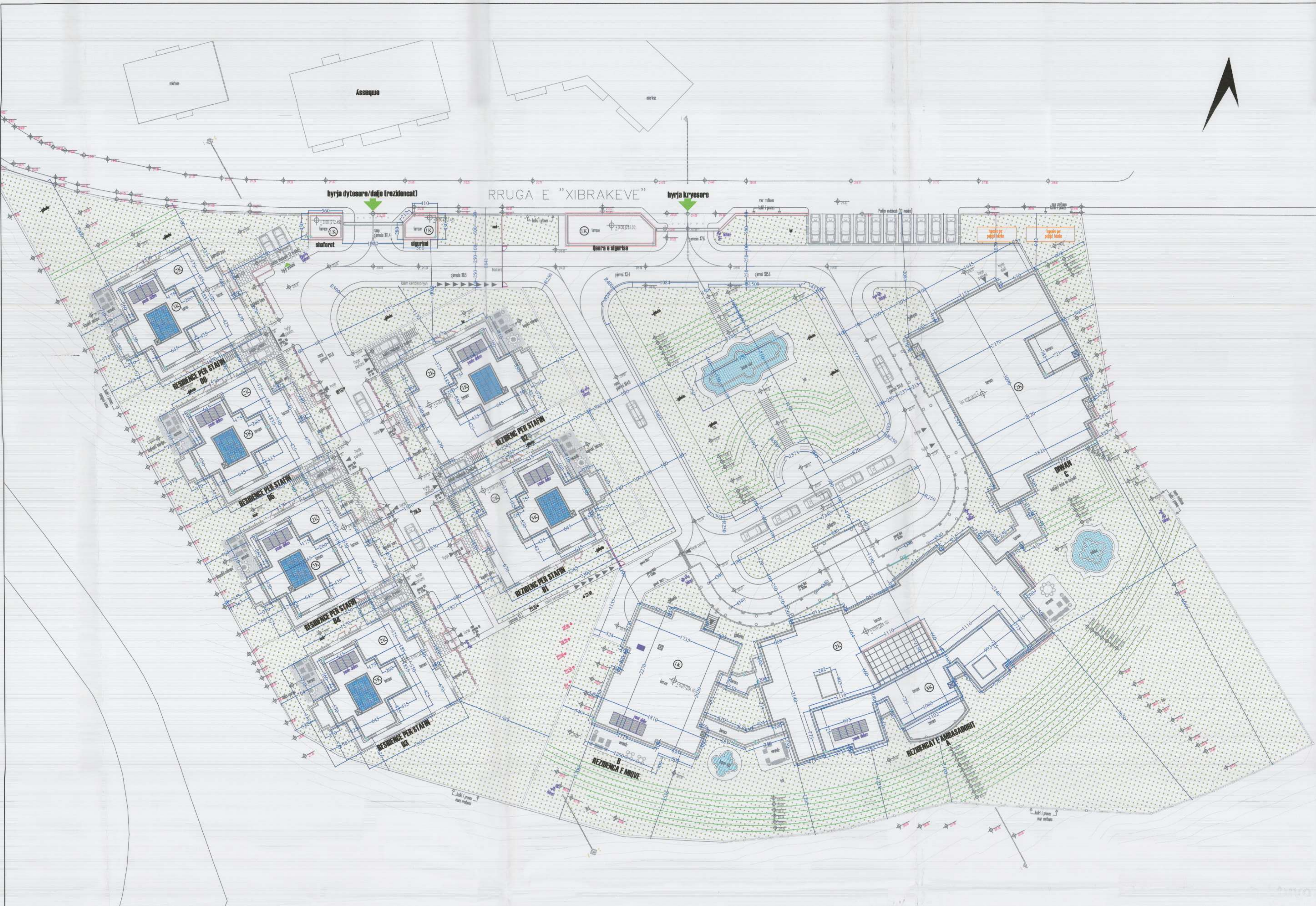
PLANI I VENDOSJES SË STRUKTURËS SHK. 1:4000
