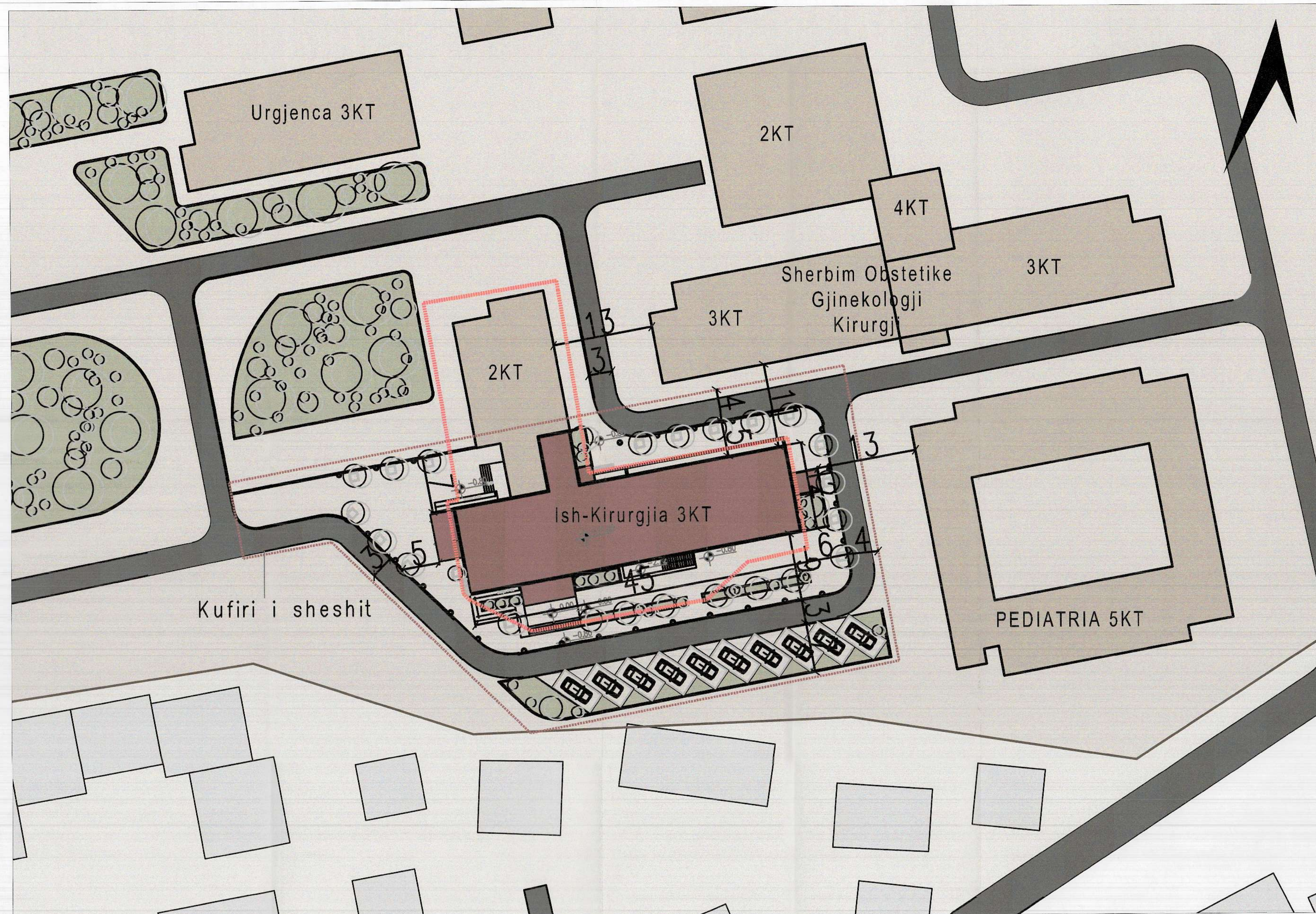
PLANI I VENDOSJES SË STRUKTURËS SHK. 1: 250
