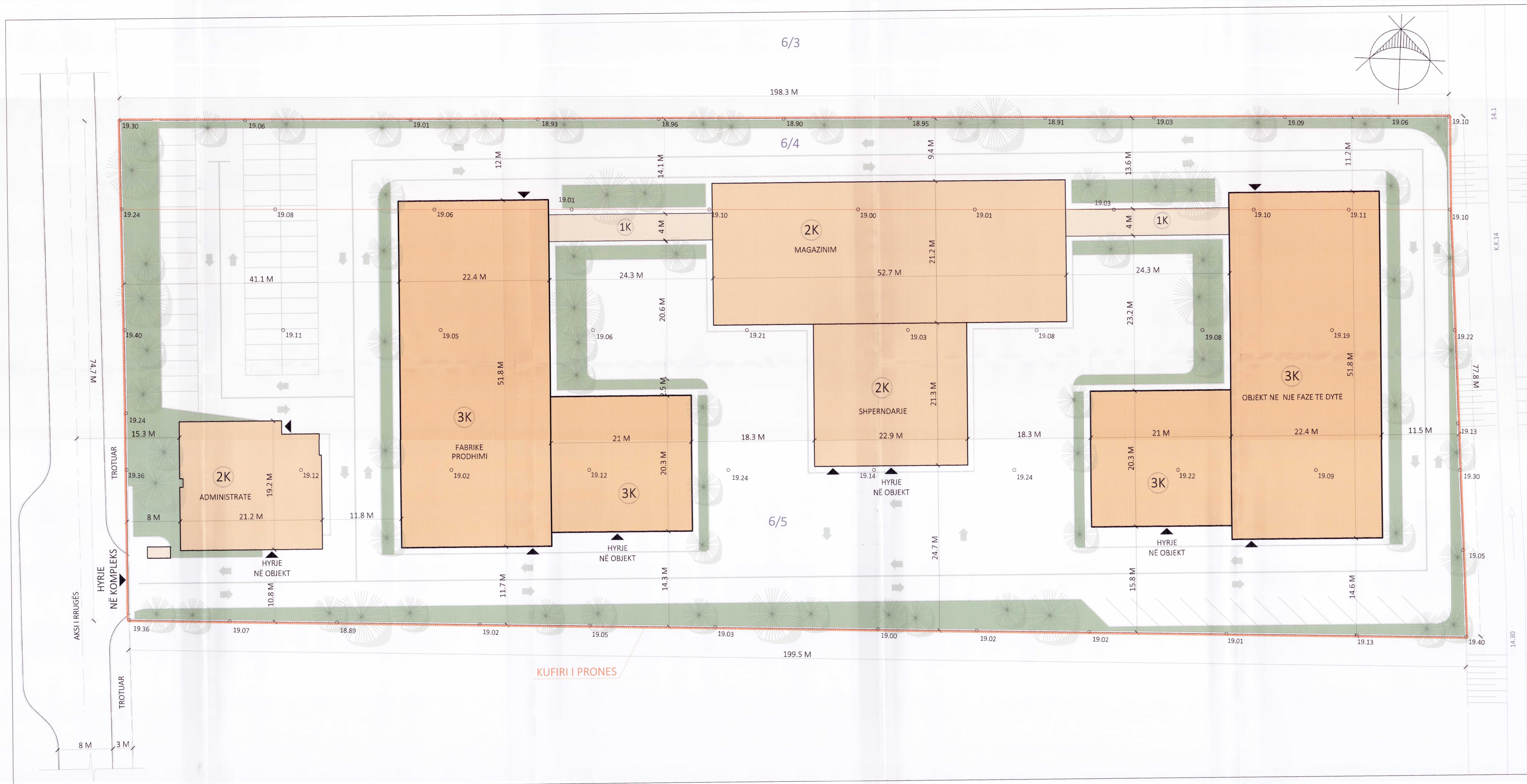
PLANI I VENDOSJES SË STRUKTURËS, SHK. 1:250
