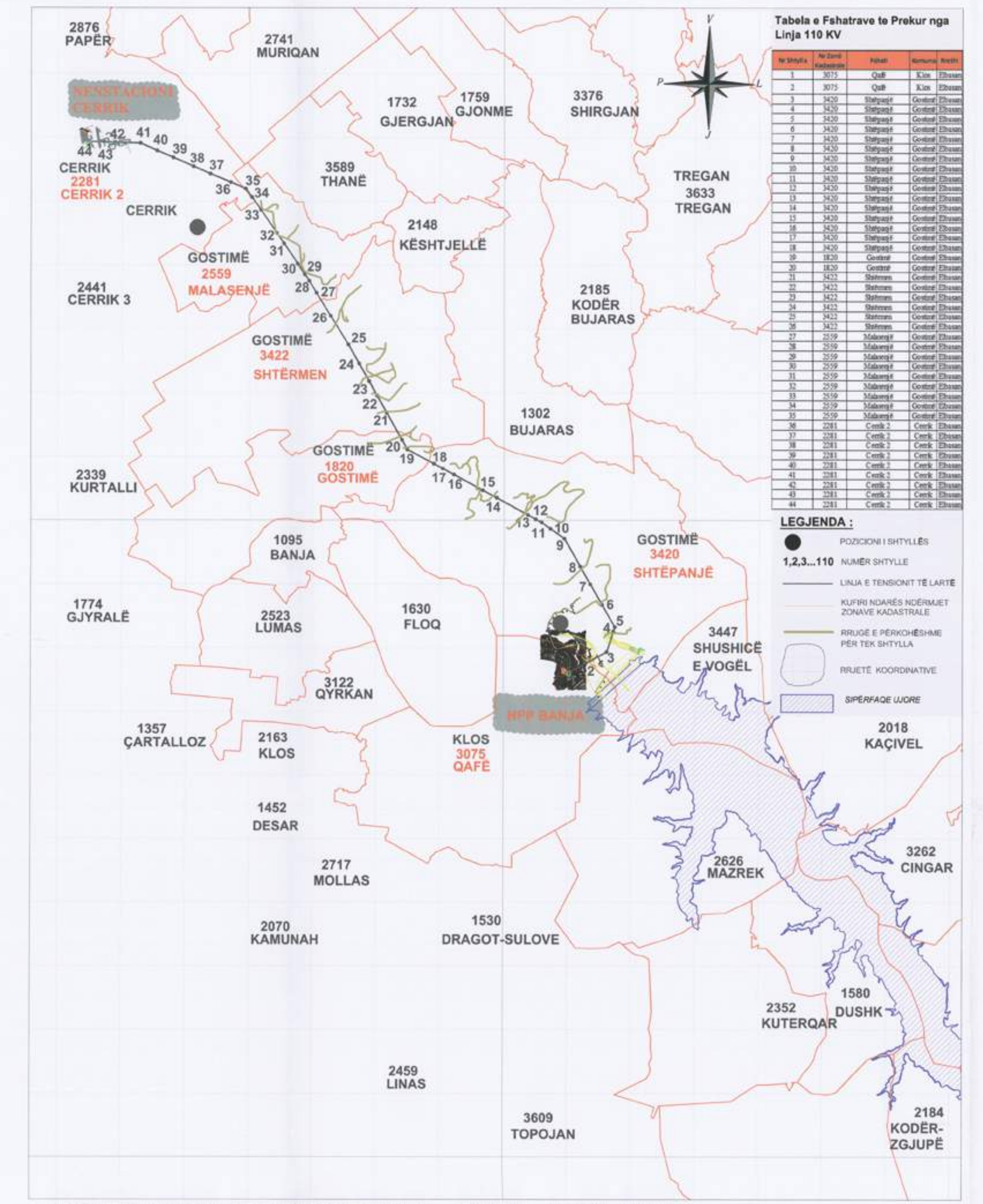
POZICIONI KADASTRAL SHK. 1:50 000
