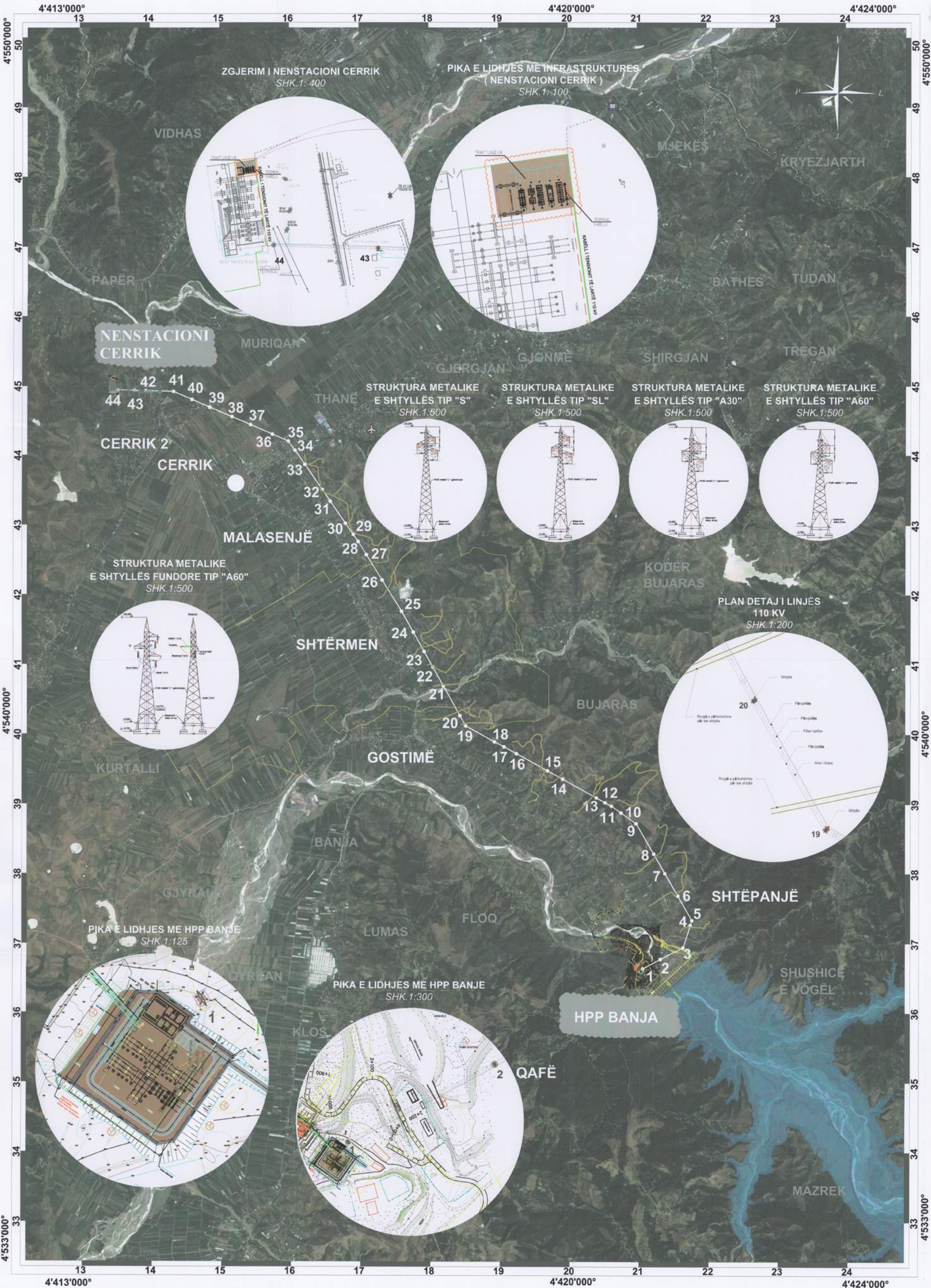
PLANI I VENDOSJES SE STRUKTURES SHK. 1: 25 000
