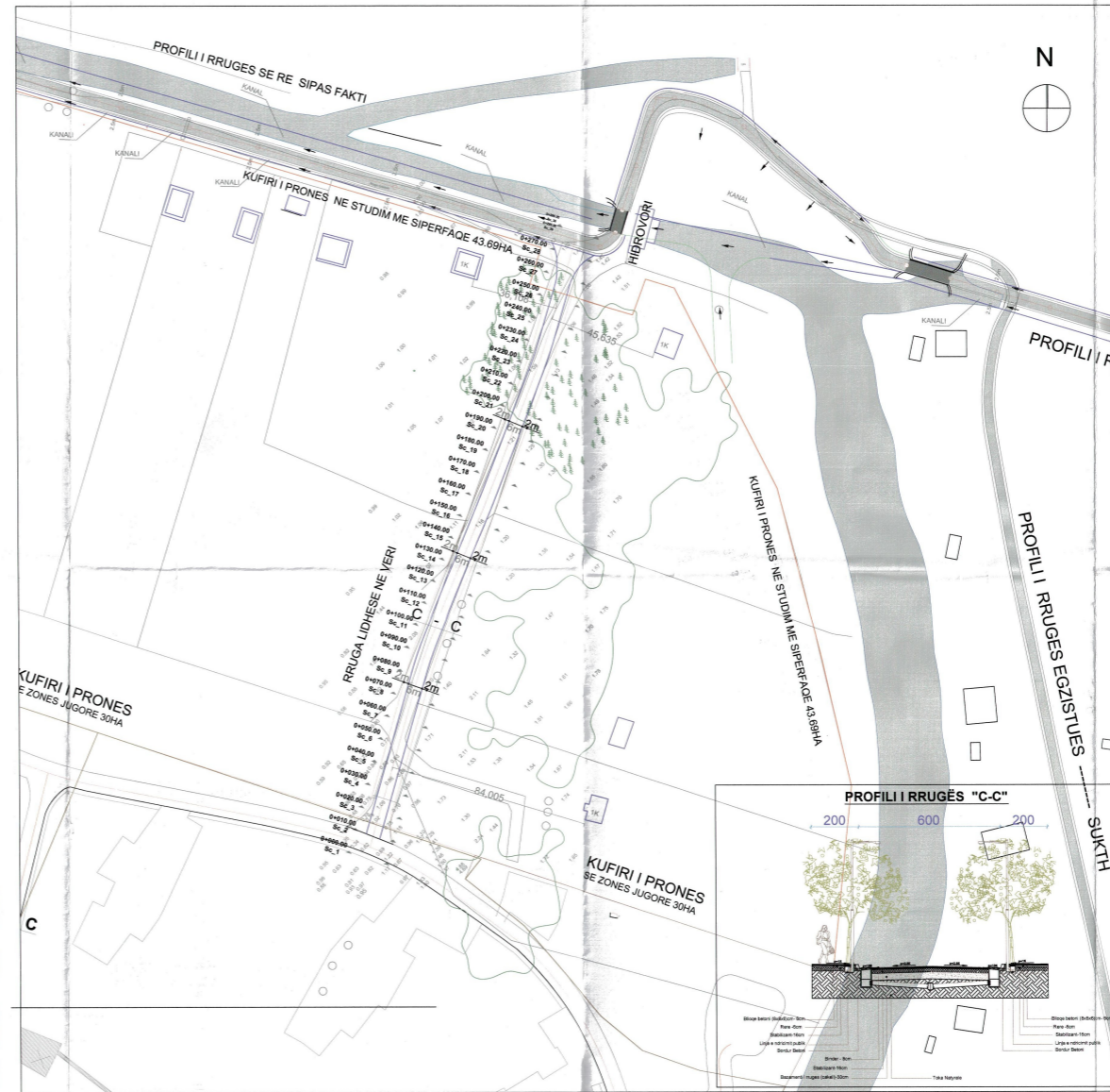
PLANI I VENDOSJES SË RRUGËS HYRËSE - DALËSE SHK. 1:1000
