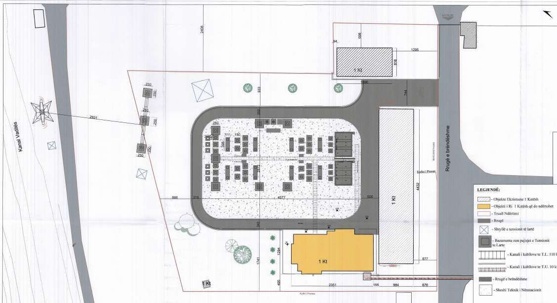
PLANI I VENDOSJES SË STRUKTURËS SHK. 1:500
