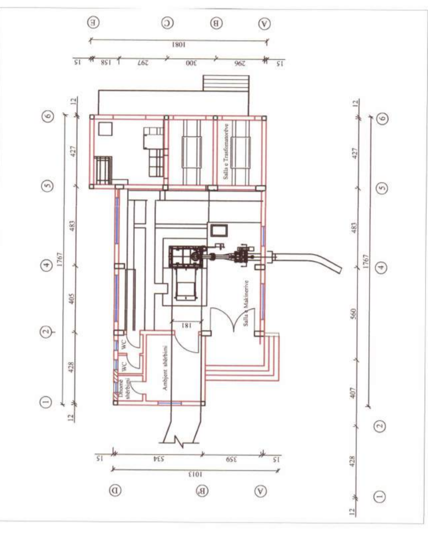
PLANIMETRIA E GODINËS SË HEC-it
