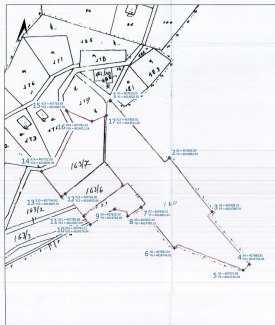
HARTA KADASTRALE E ZONES SHK. 1: 1500
