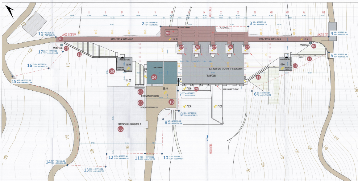
PLANI I VENDOSJES SE STRUKTURES SHK 1:350
