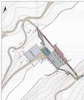
RILEVIMI TOPOGRAFIK I ZONES SHK. 1: 1500
