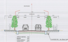
PROFIL TIP SHK. 1:100
