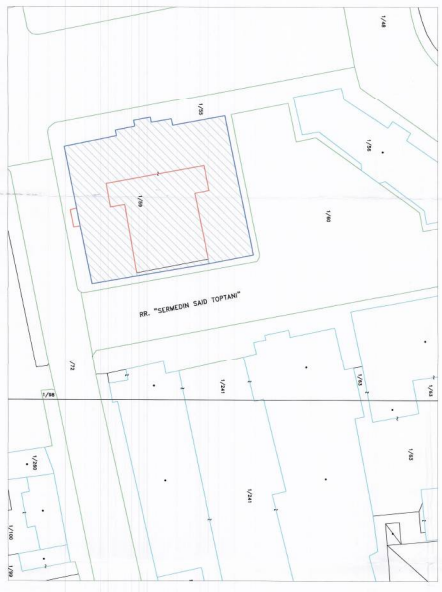
POZICIONI KADASTRAL TR.P-11 SH.K. 1:500
