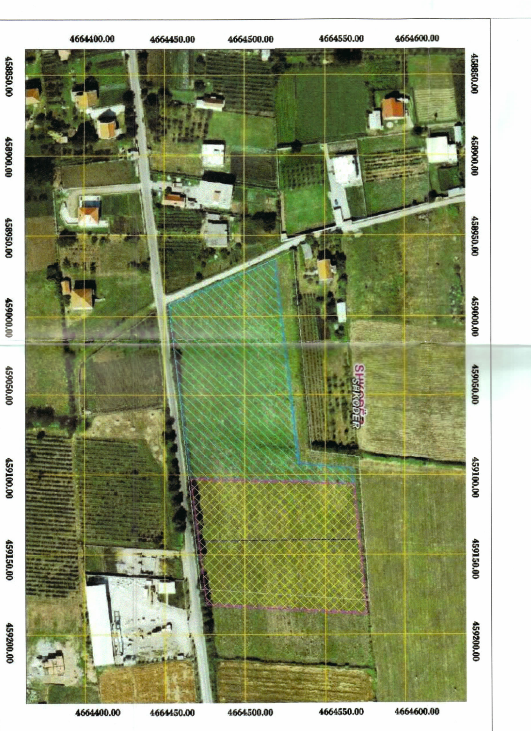
HARTA TOPOGRAFIKE SHK. 1:1000
