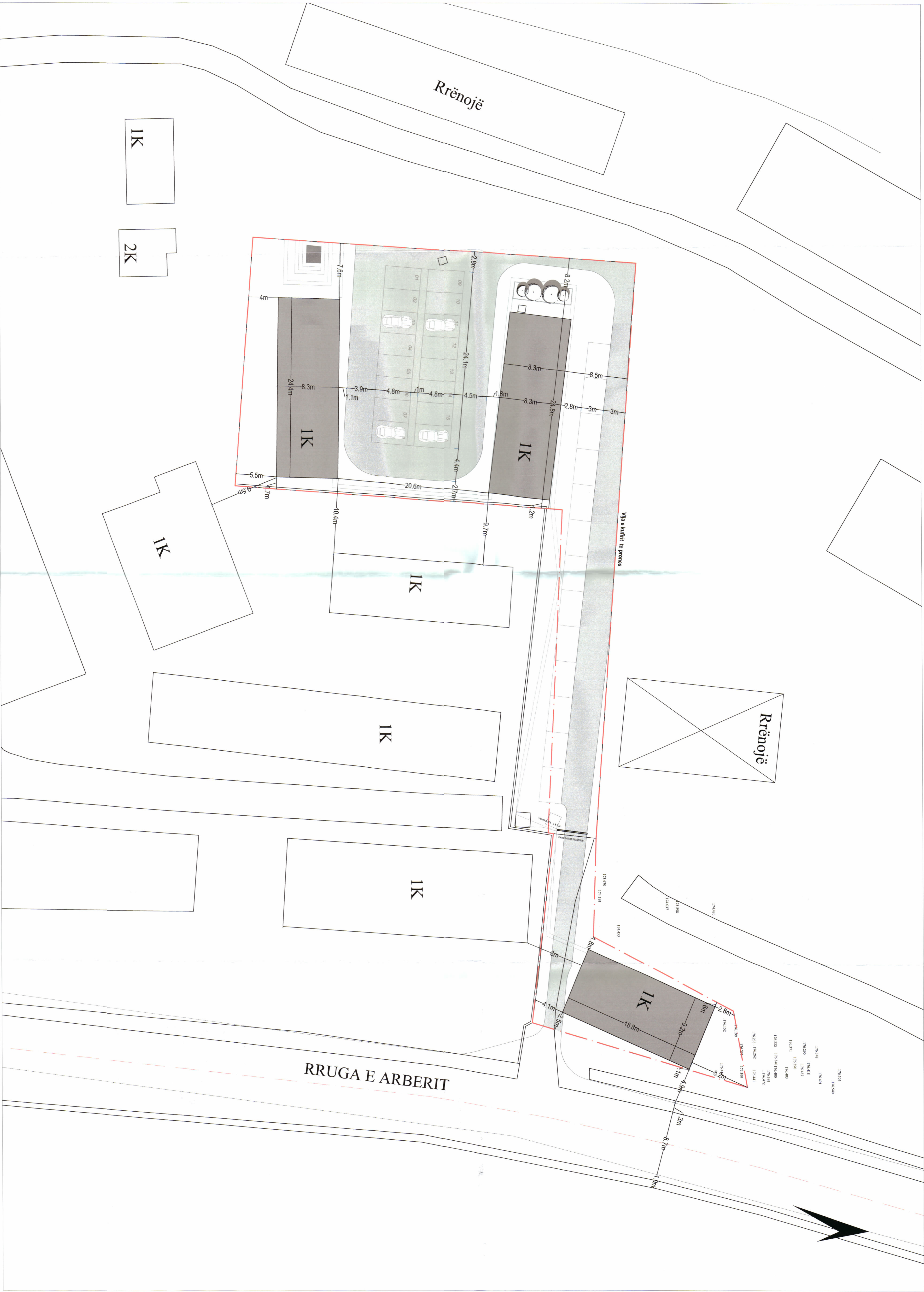
PLANI I VENDOSIES SË STRUKTURËS SHK. 1: 250
