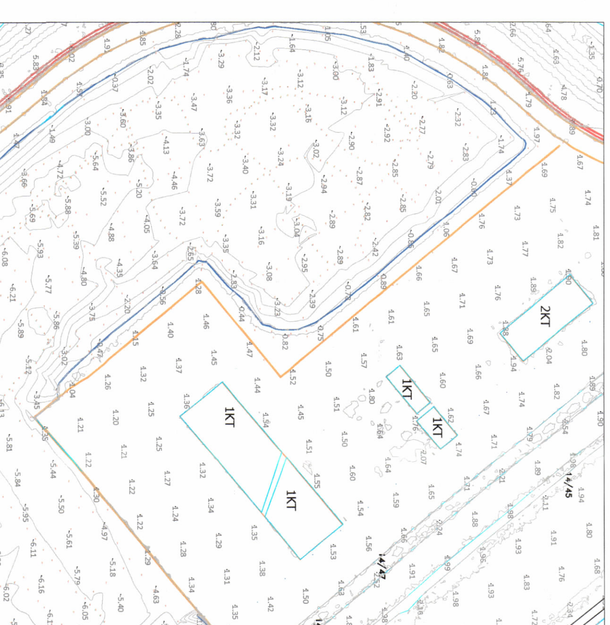
HARTA TOPOGRAFIKE SHK. 1:1000
