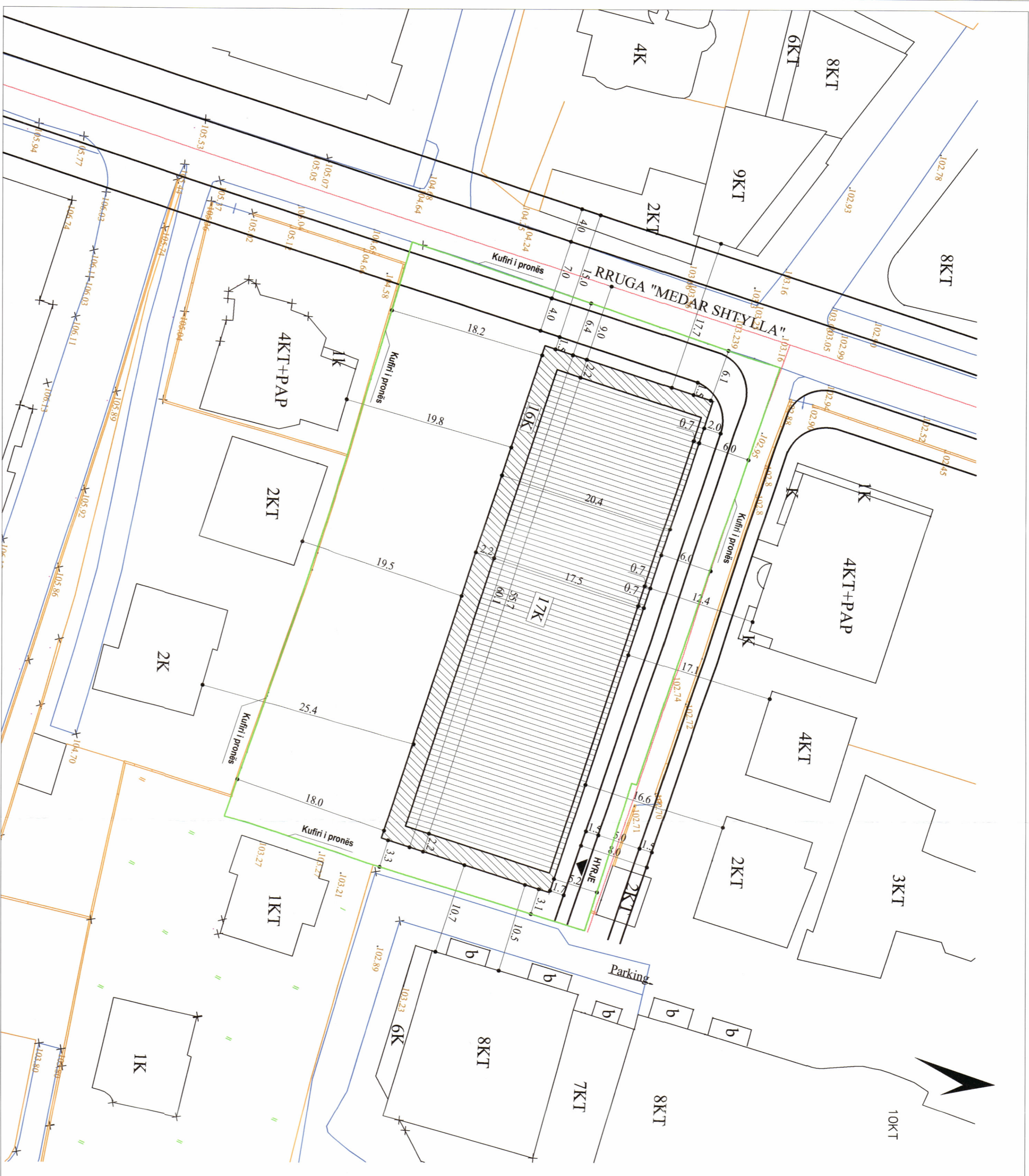
PLANI I VENDOSIES SË STRUKTURES SHK. 1: 500
