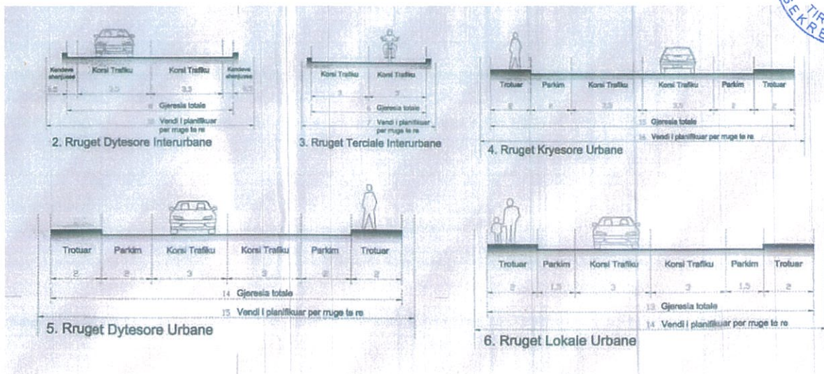
Fig.3 Fragment i hartës së rrjetit rrugor të propozuar _Seksionet e rrugeve
