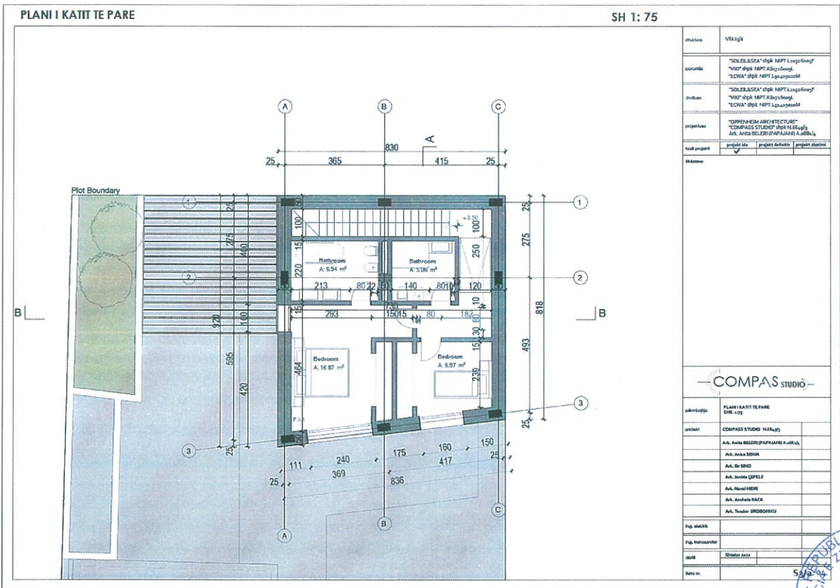
Fig.12 Vila S3/a _ Planimetria e katit të parë
