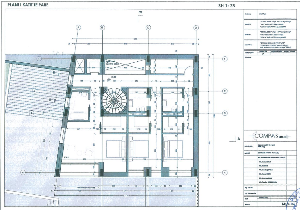
Fig.34 Vila M3/a _Planimetria e katit të parë
