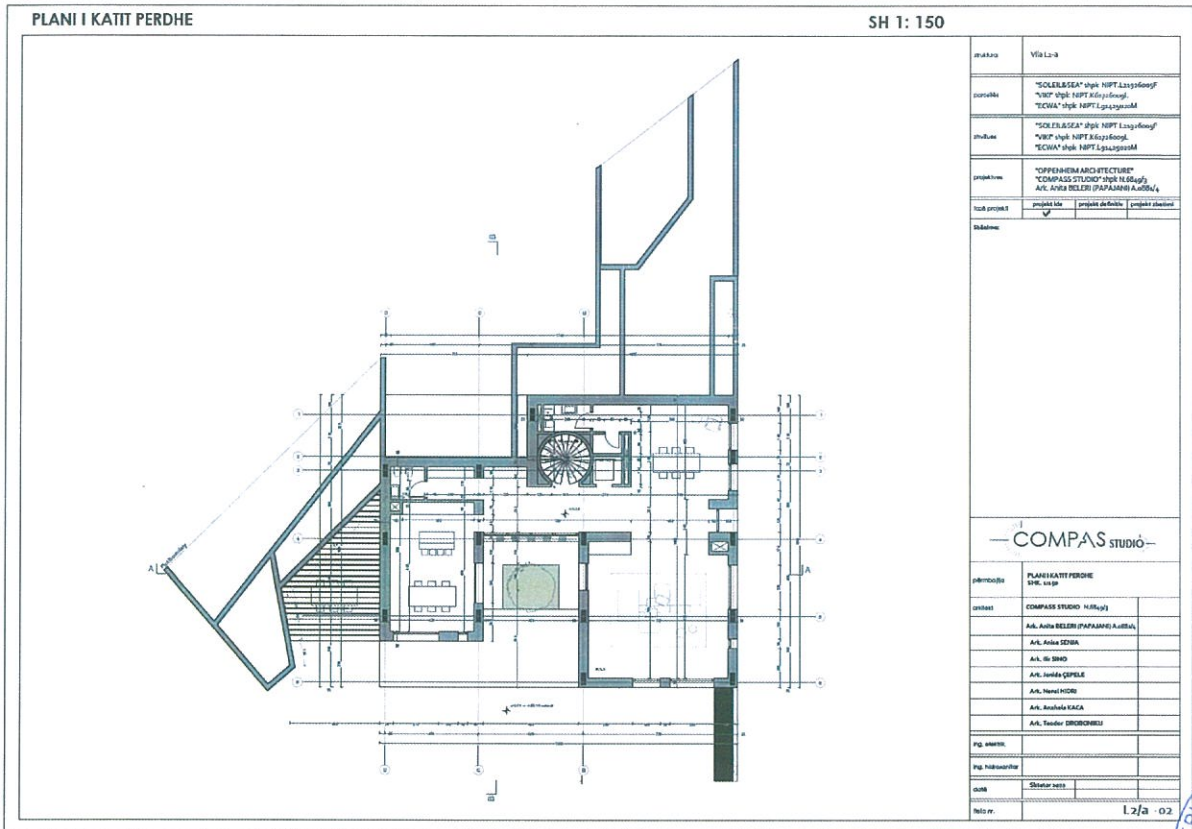
Fig.44 Vila L2-a _ Planimetria e katit përdhe
