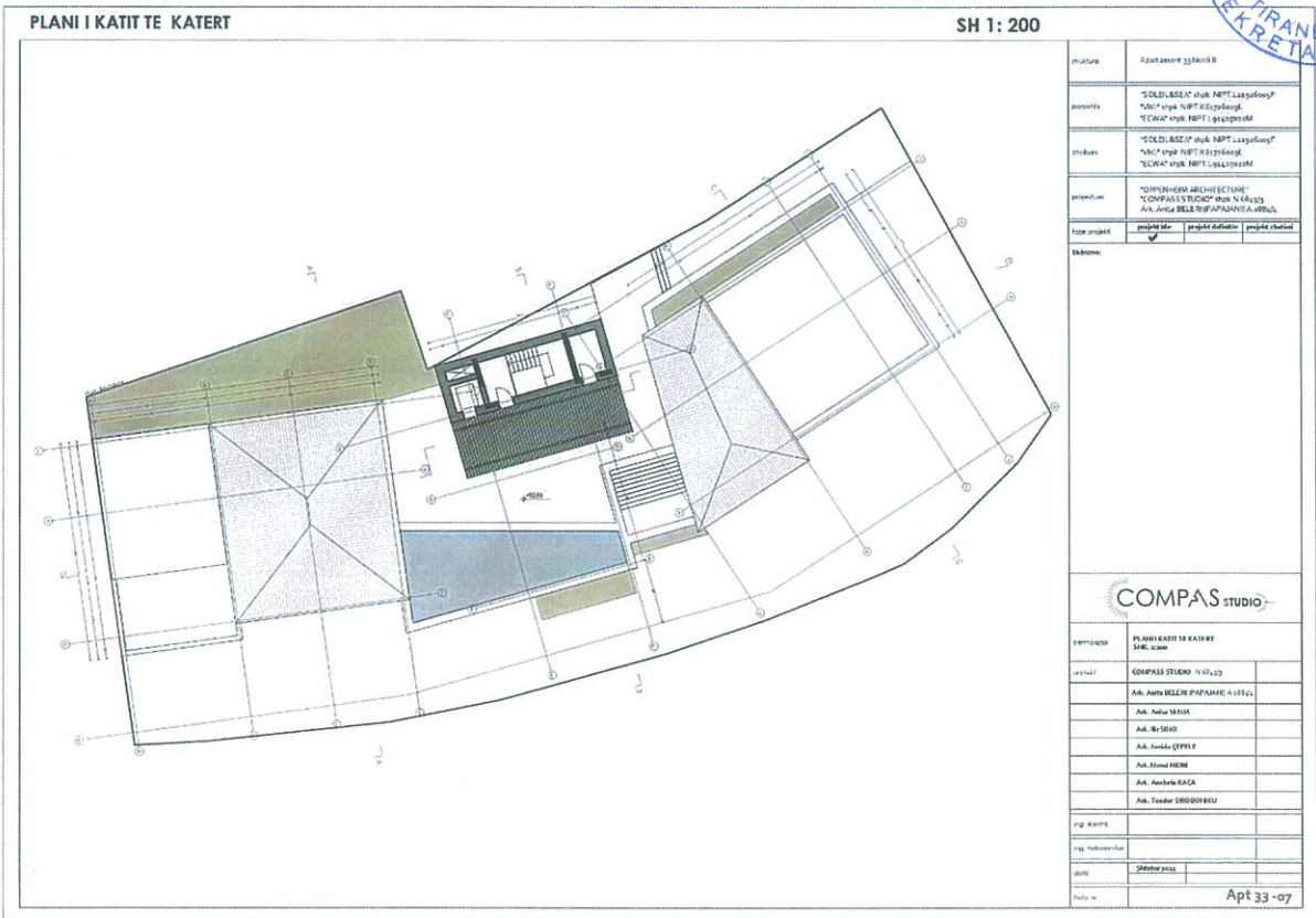
Fig.78 Objekti 33_Planimetria e katit të katërt
