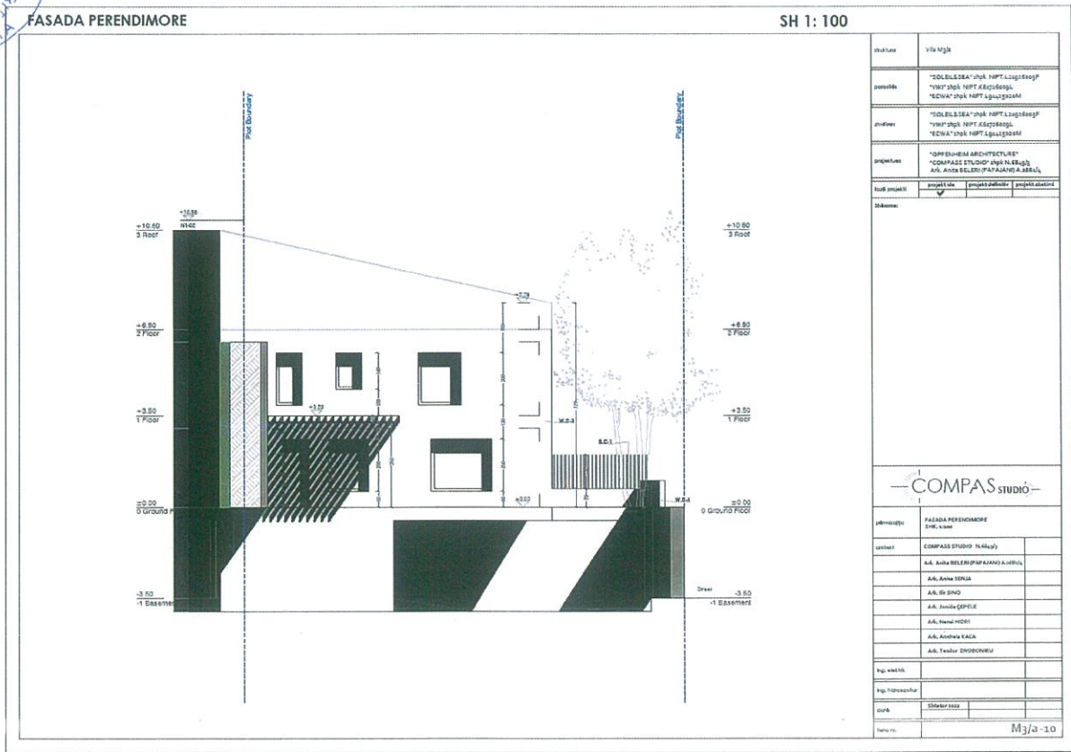
Fig.40 Vila M3/a _ Fasada Perendimore
