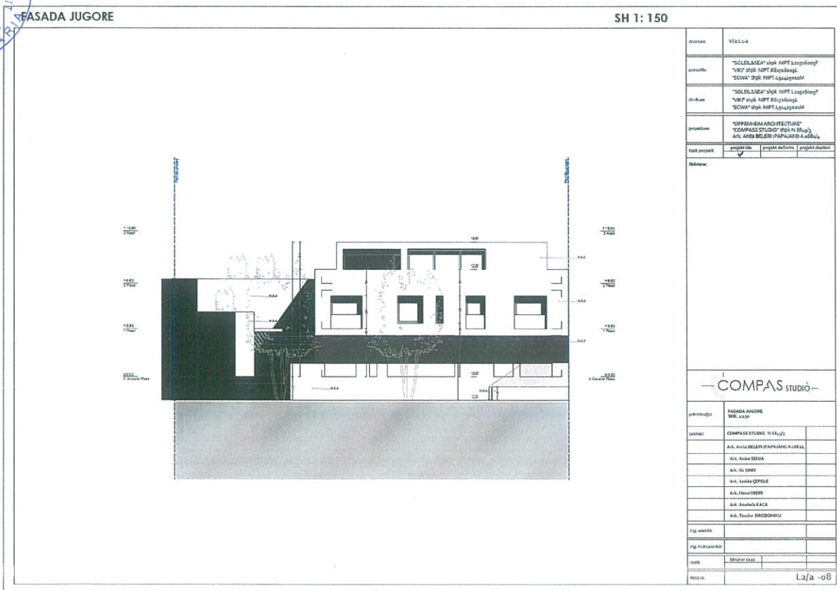
Fig.50 Vila L2-a _ Fasada Jugore
