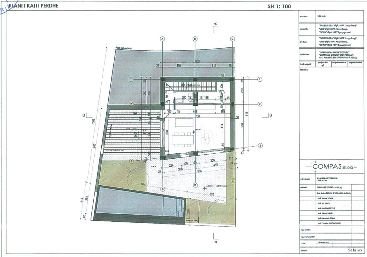
Fig.21 Vila S2/a _ Planimetria e katit përdhe
