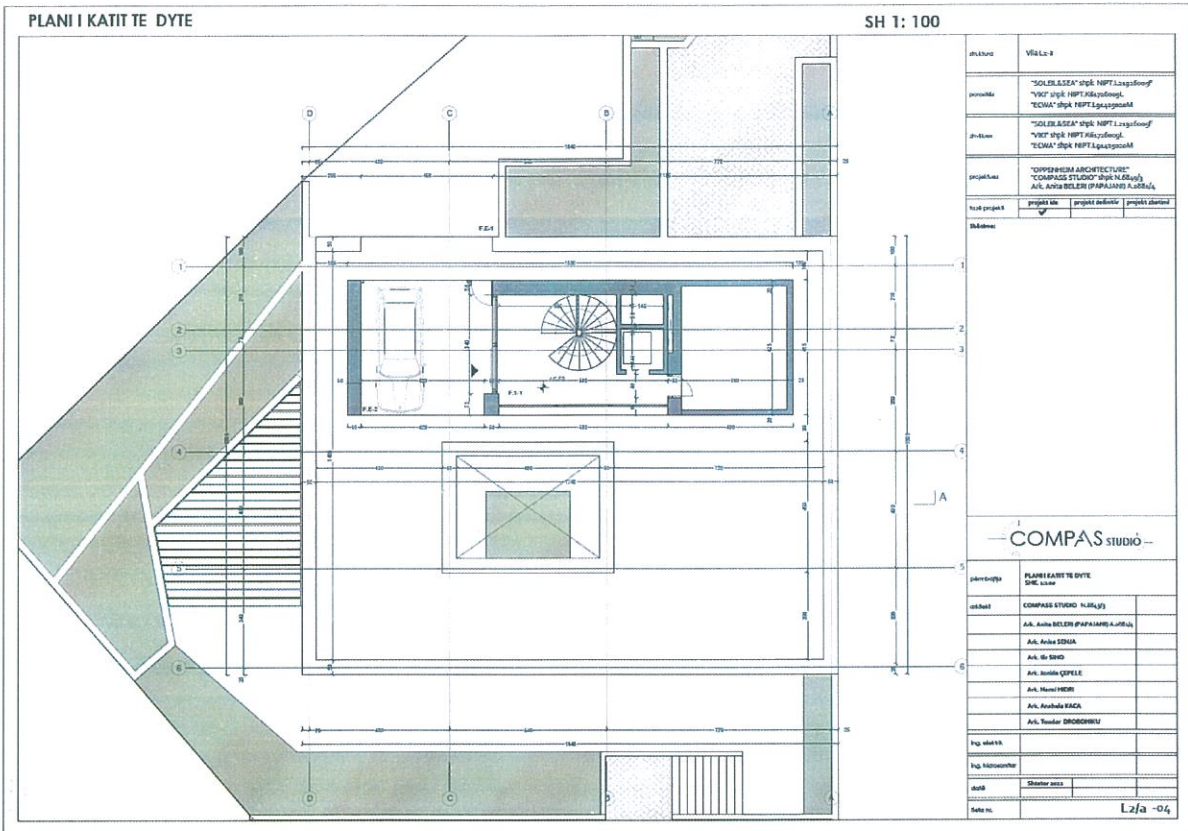
Fig.46 Vila L2-a _Planimetria e katit të dytë
