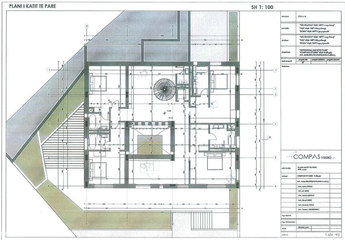
Fig.45 Vila L2-a _ Planimetria e katit të parë
