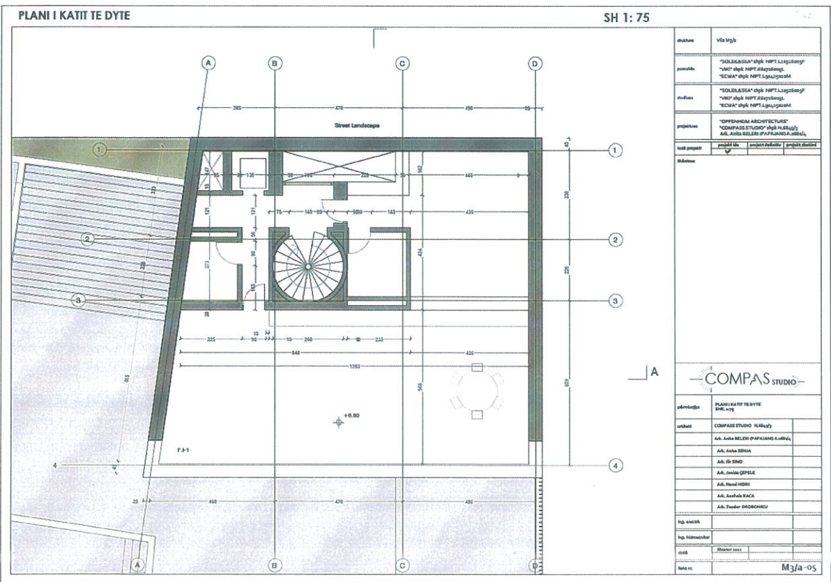
Fig.35 Vila M3/a _Planimetria e katit të dytë
