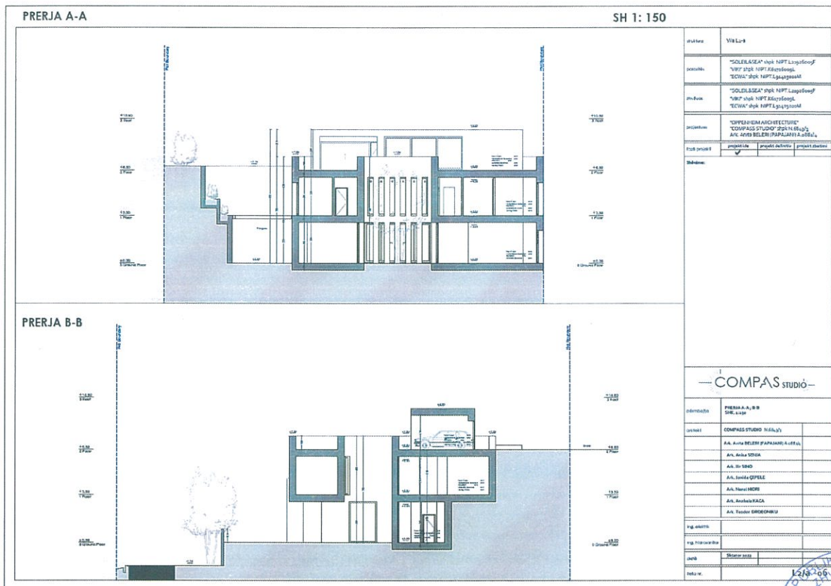
Fig.48 Vila L2-a _Prerjet
