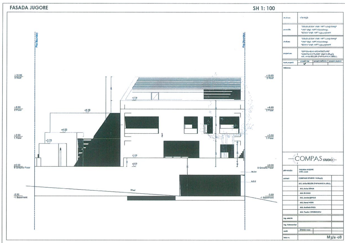
Fig.38 Vila M3/a _ Fasada Jugore
