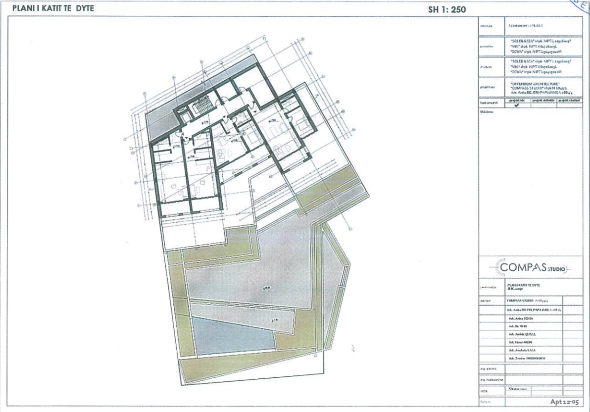
Fig.60 Objekti 12_Planimetria e katit të dytë
