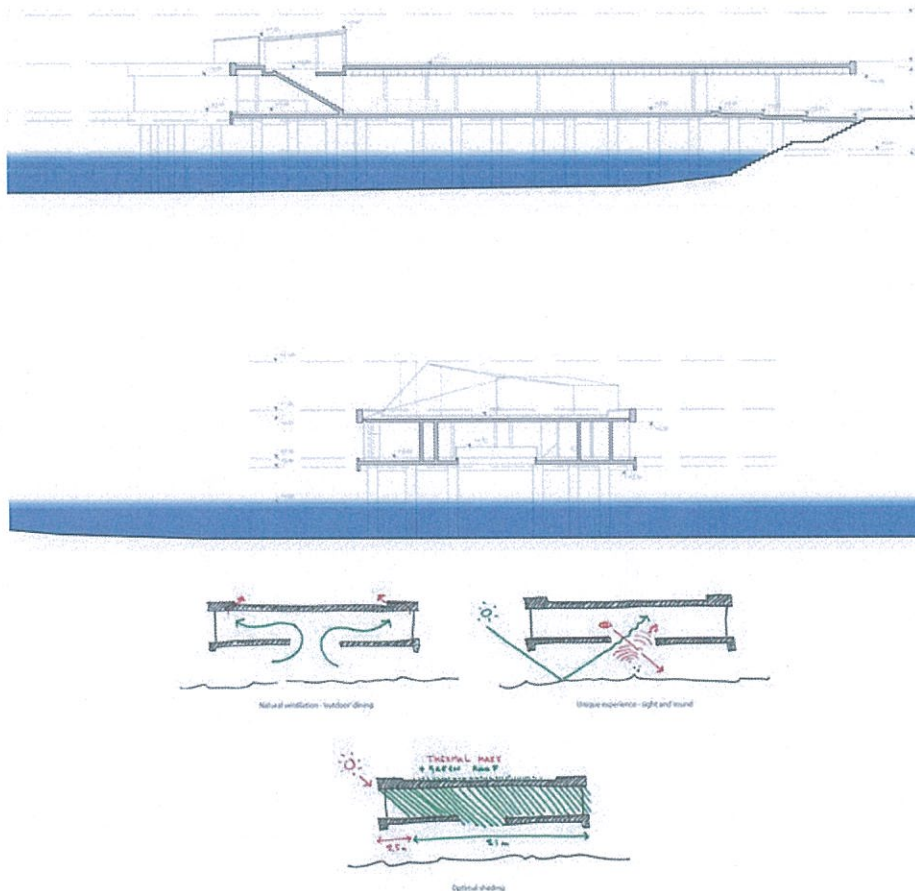
Fig. 6. Skema e objektit ne altimetri
