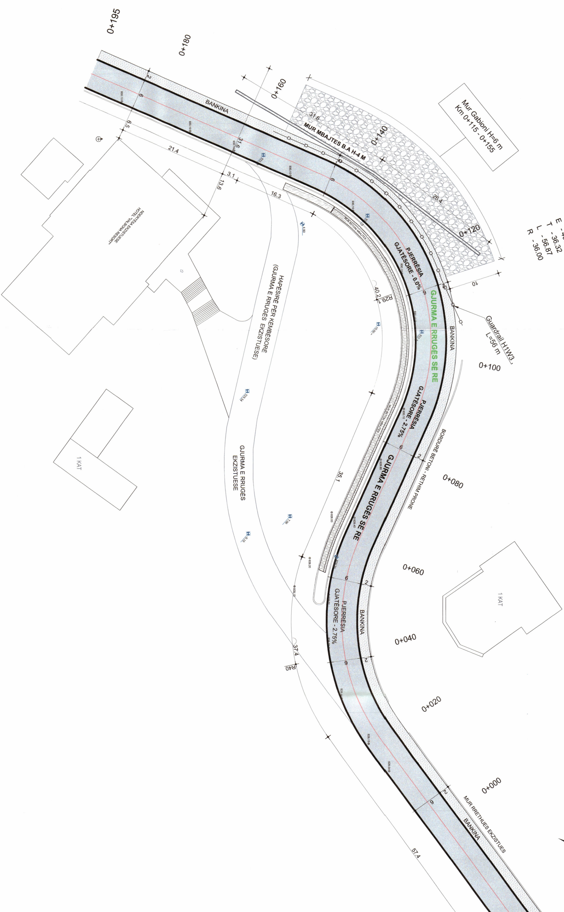
PLANI I VENDOSJES SË STRUKTURËS SHK. 1: 250
