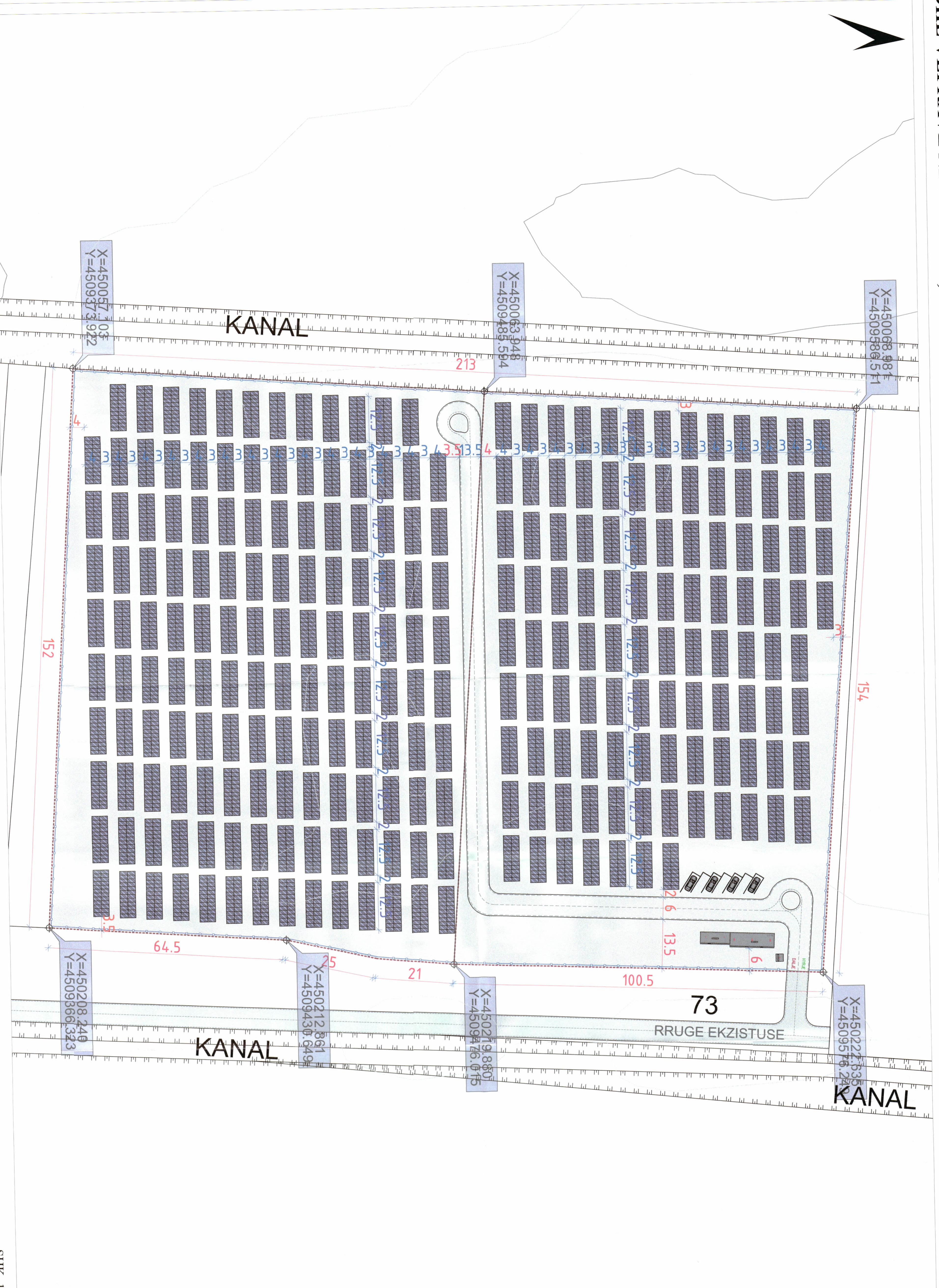
PLANI I VENDOSIES SË STRUKTURËS
