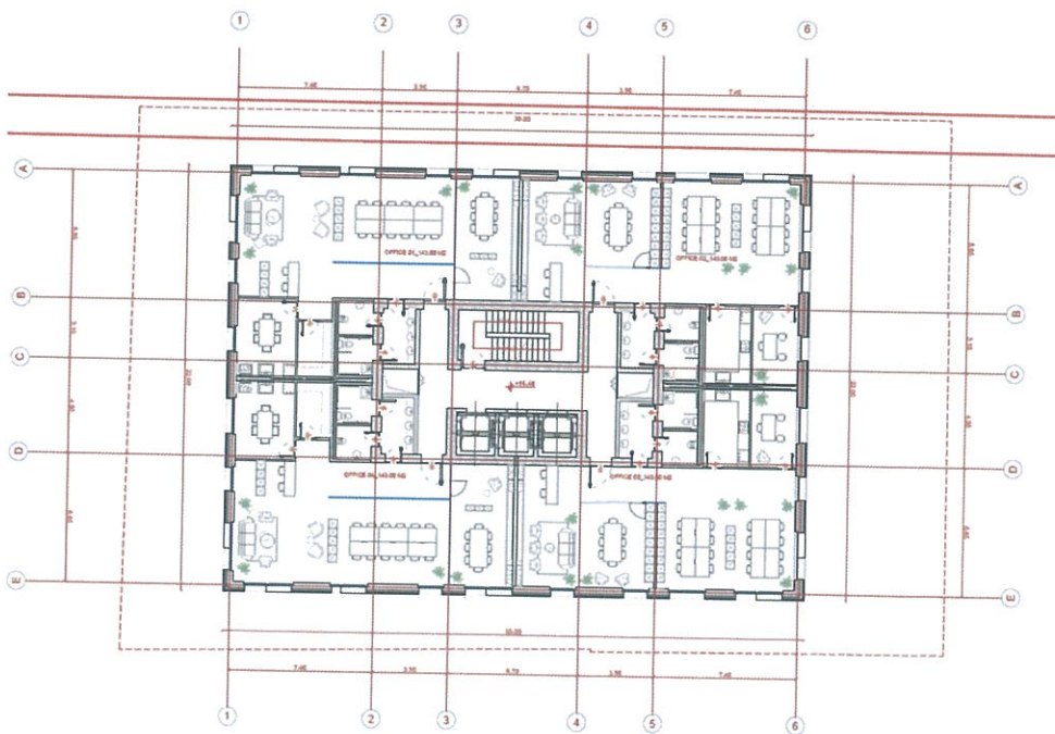
Fig.7 Planimetria e kateve te zyrave
