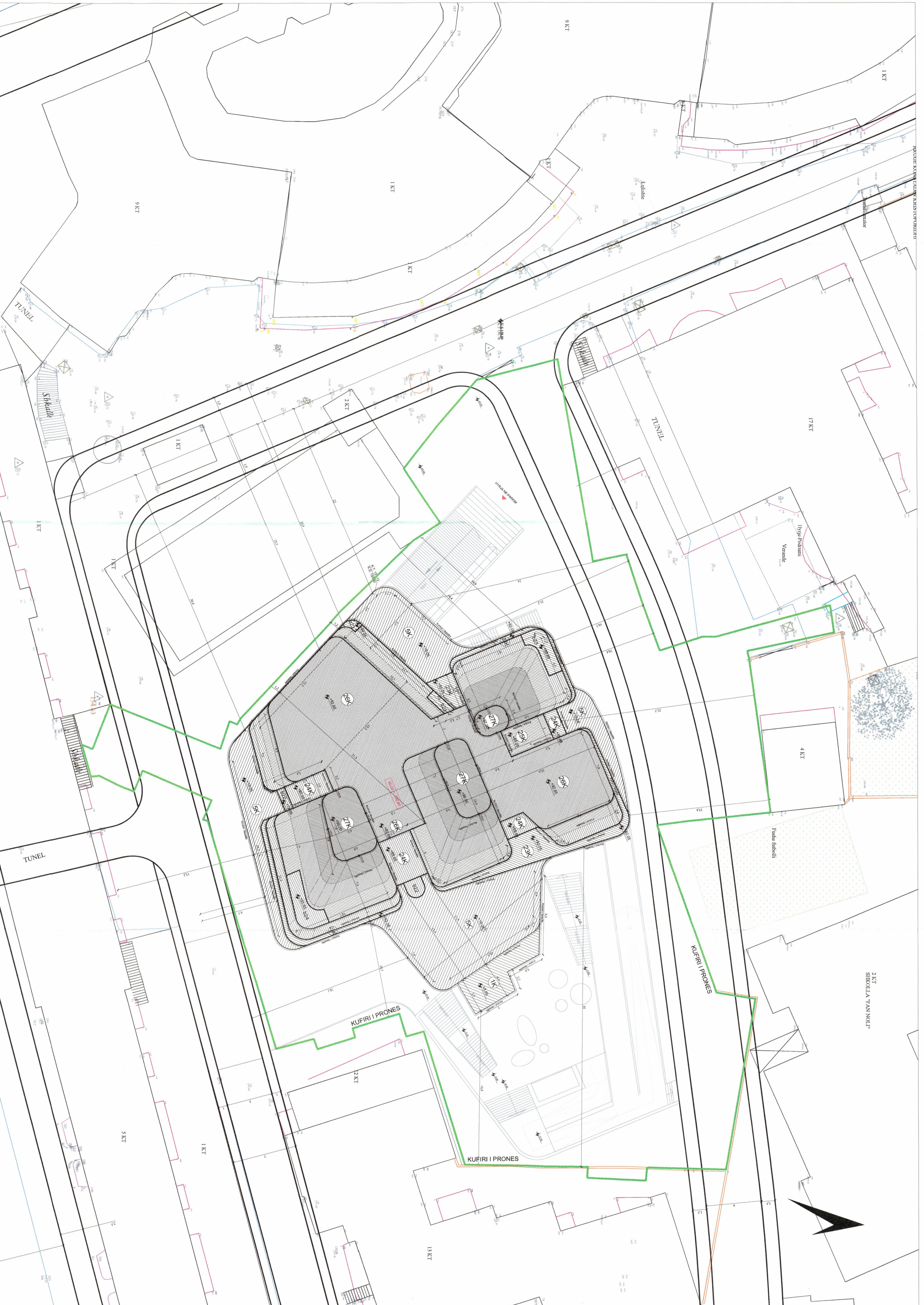
PLANI I VENDOSJES SË STRUKTURËS SHK. 1: 200
