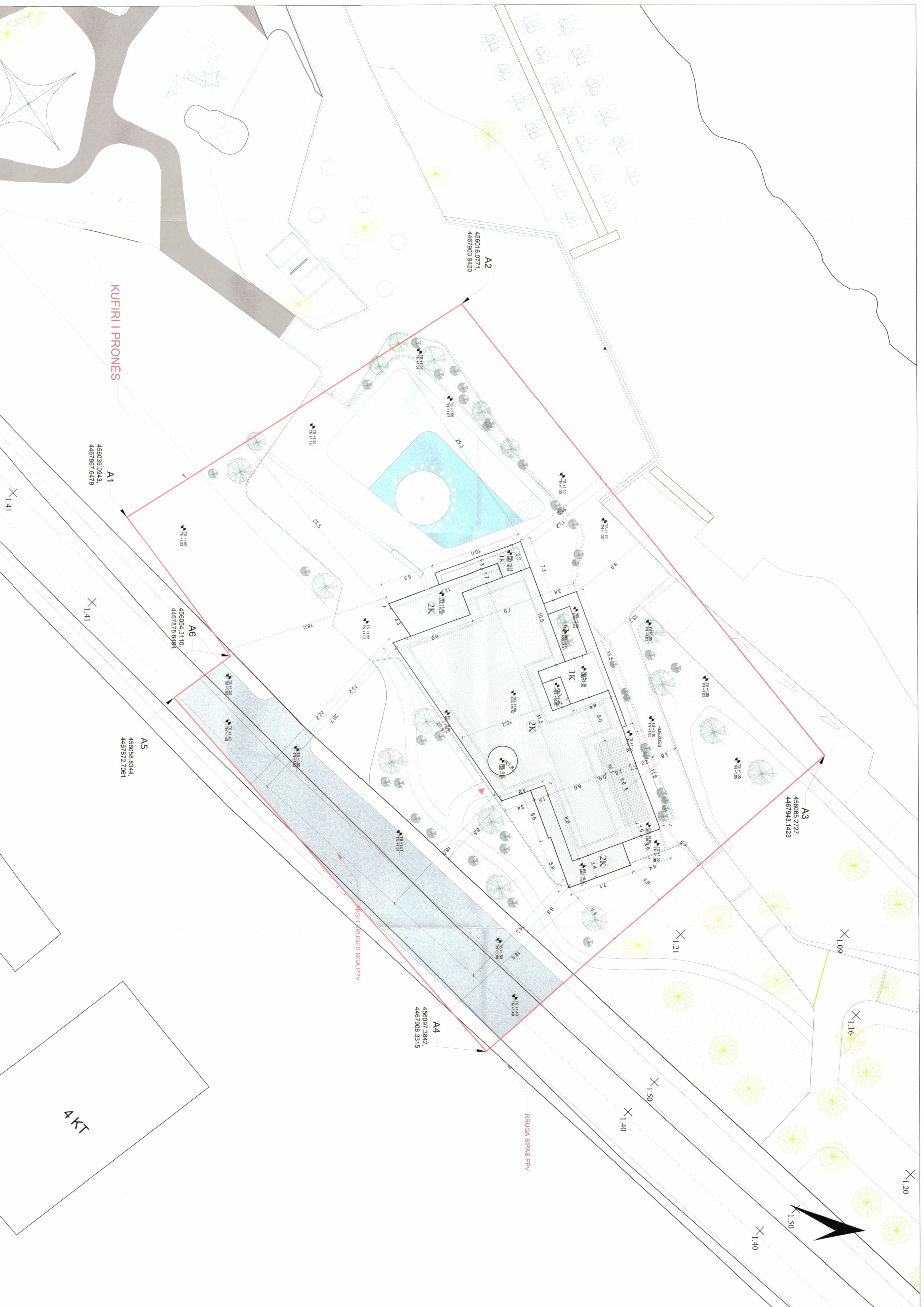
PLANI I VENDOSIES SË STRUKTURËS SHK. 1:200
