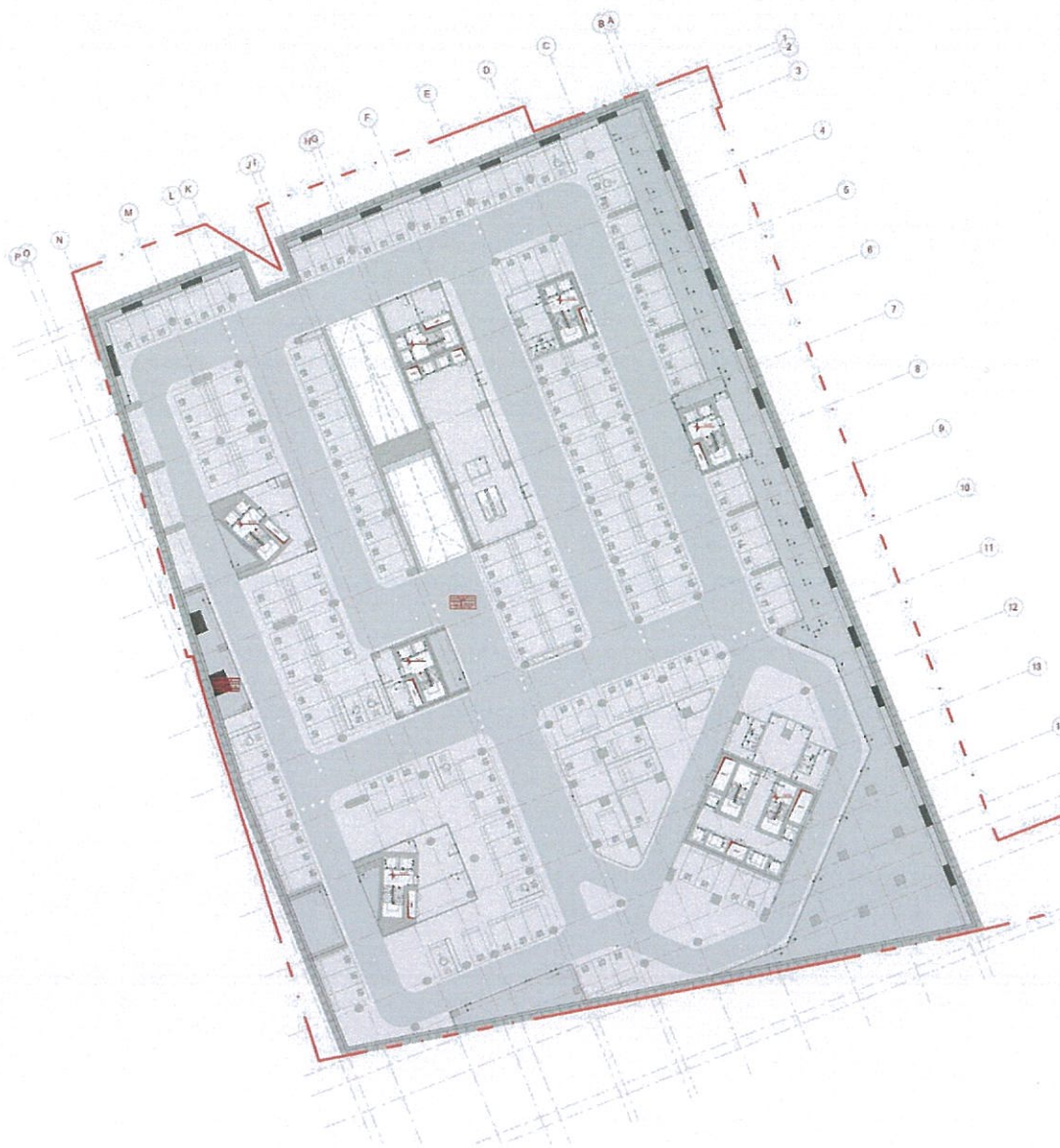
Fig. 12. Skemë shpjeguese organizimit të Katit të Dytë Nëntokësor.
