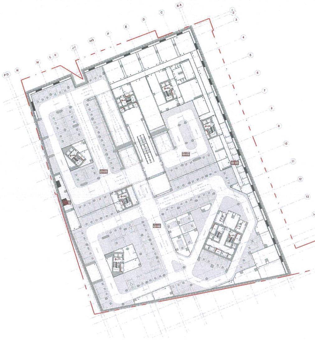
Fig. 11. Skemë shpjeguese e organizimit të Katit të Parë Nëntokësor.
