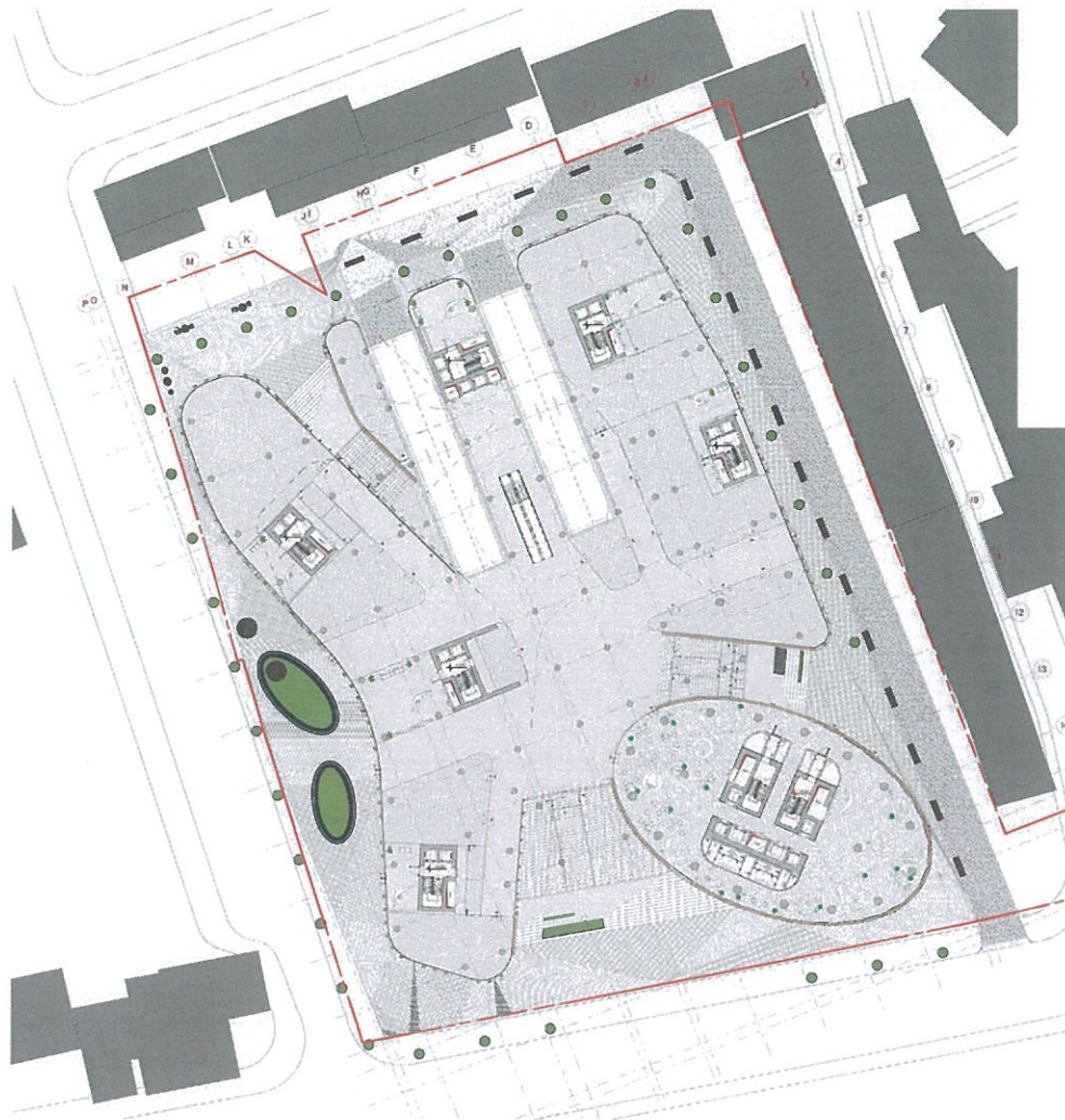
Fig. 9. Skemë shpjeguese organizimi në Katin Përdhe.
