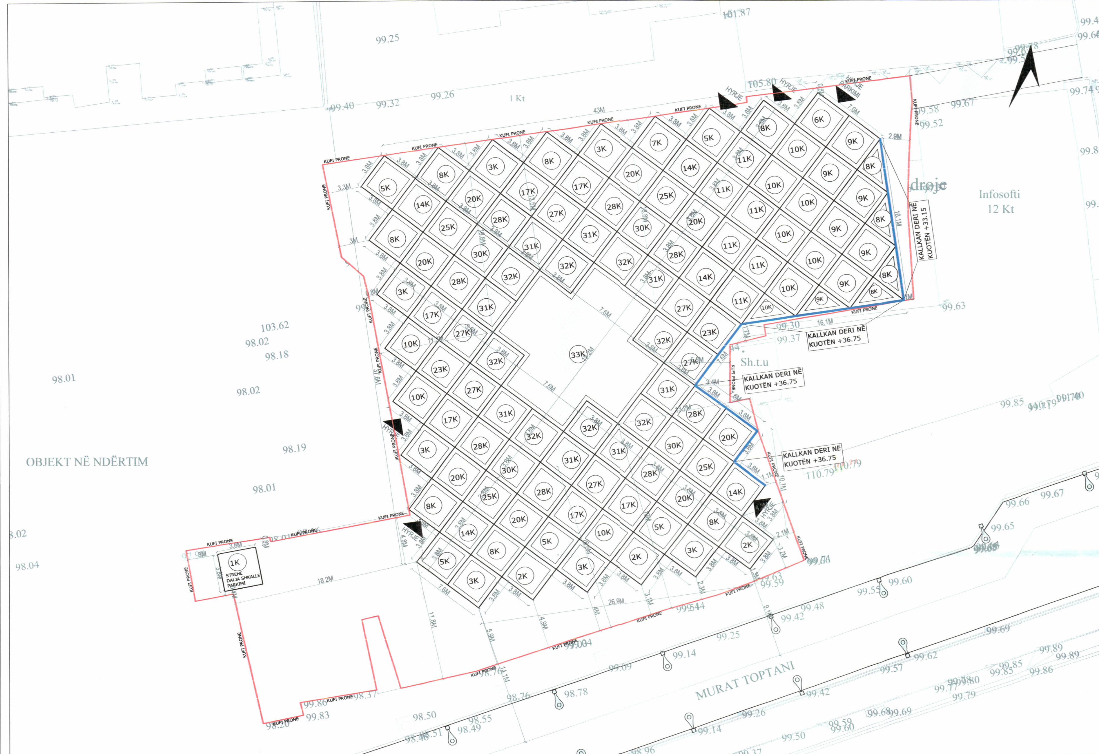
PLANI I VENDOSJES SË STRUKTURËS SHK. 1: 150
