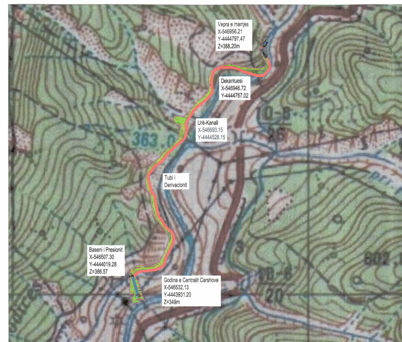
HARTA TOPOGRAFIKE SHK. 1:7500
