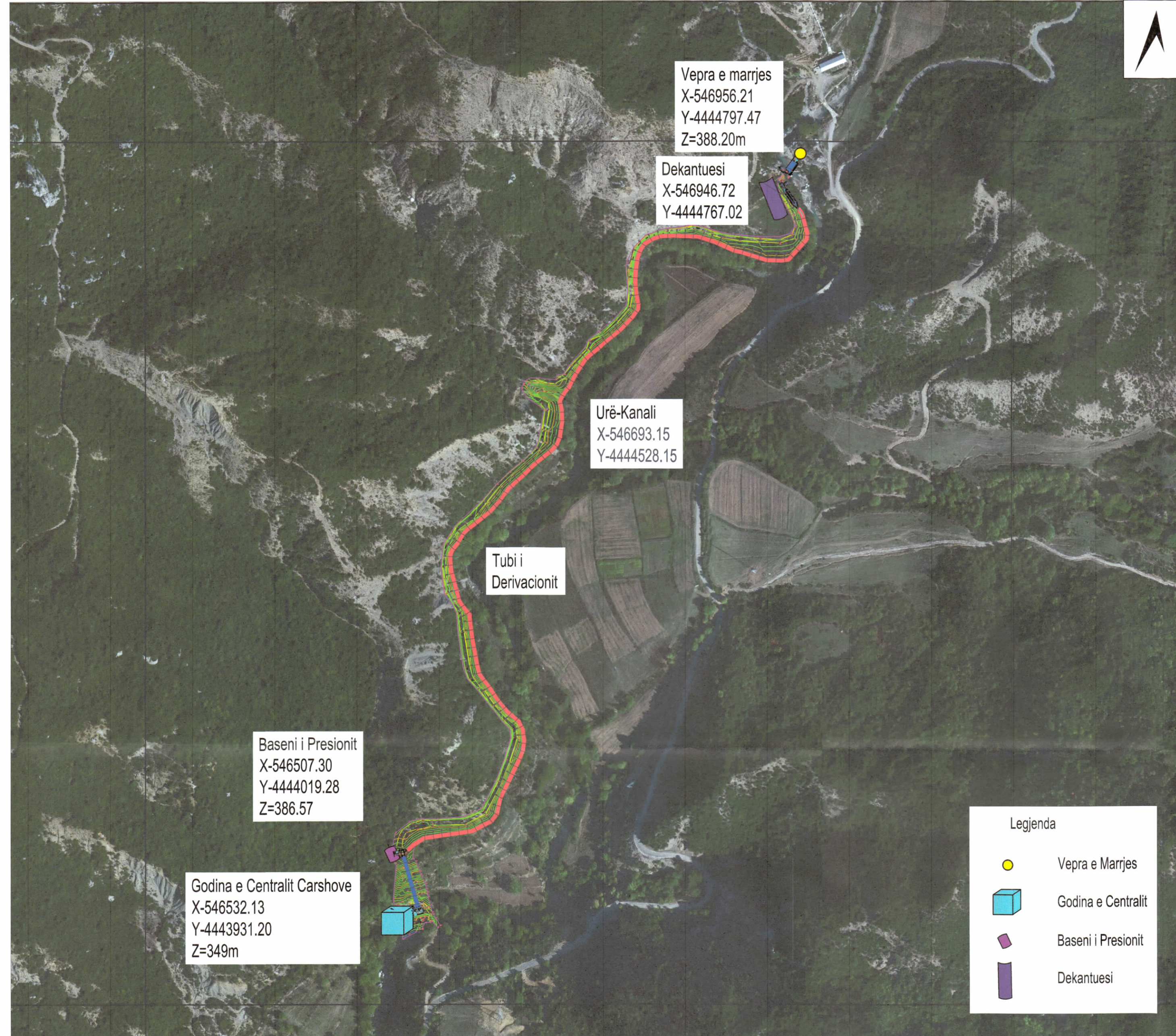
PLANI I VENDOSJES SË STRUKTURËS SHK. 1: 3500
