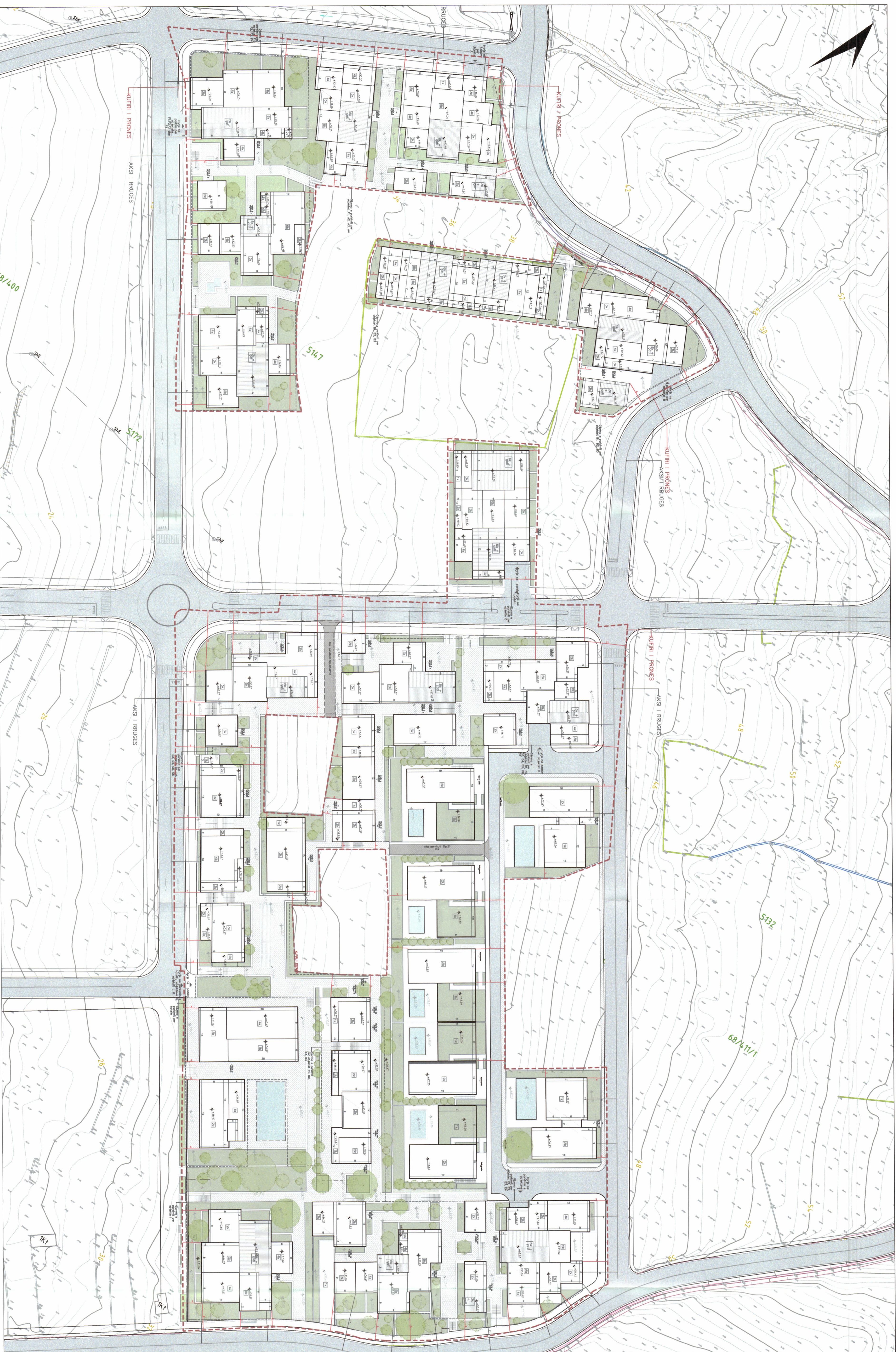
PLANI I VENDOSIES SË STRUKTURËS SHK. 1: 500
