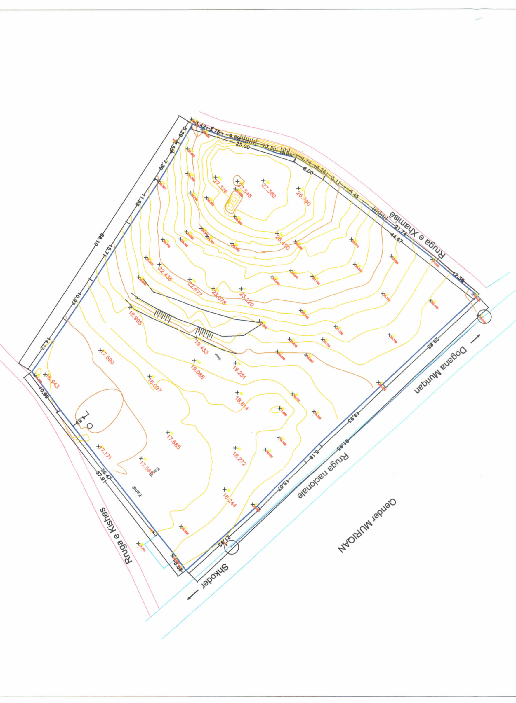
HARTA TOPOGRAFIKE SHK. 1:500
