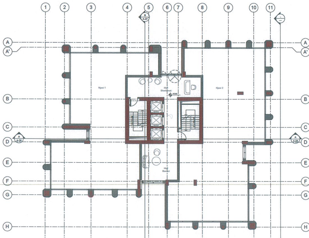
Fig. 9 – Plani i Katit Përdhe - Shërbim, Kuota +0.00
