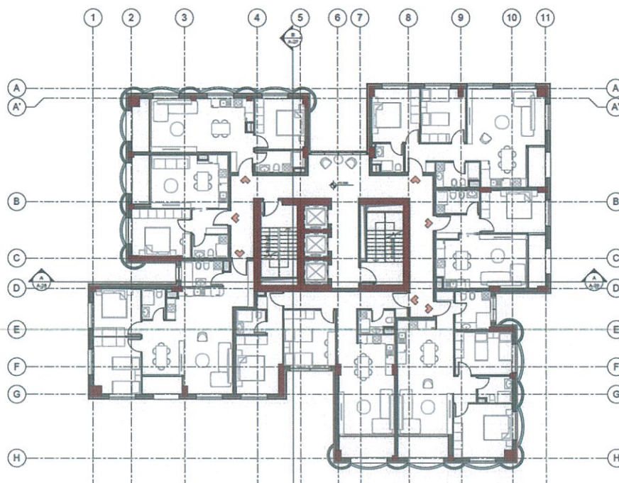
Fig. 11 – Plani i Katit +8 – Banim, Kuota +31.68
