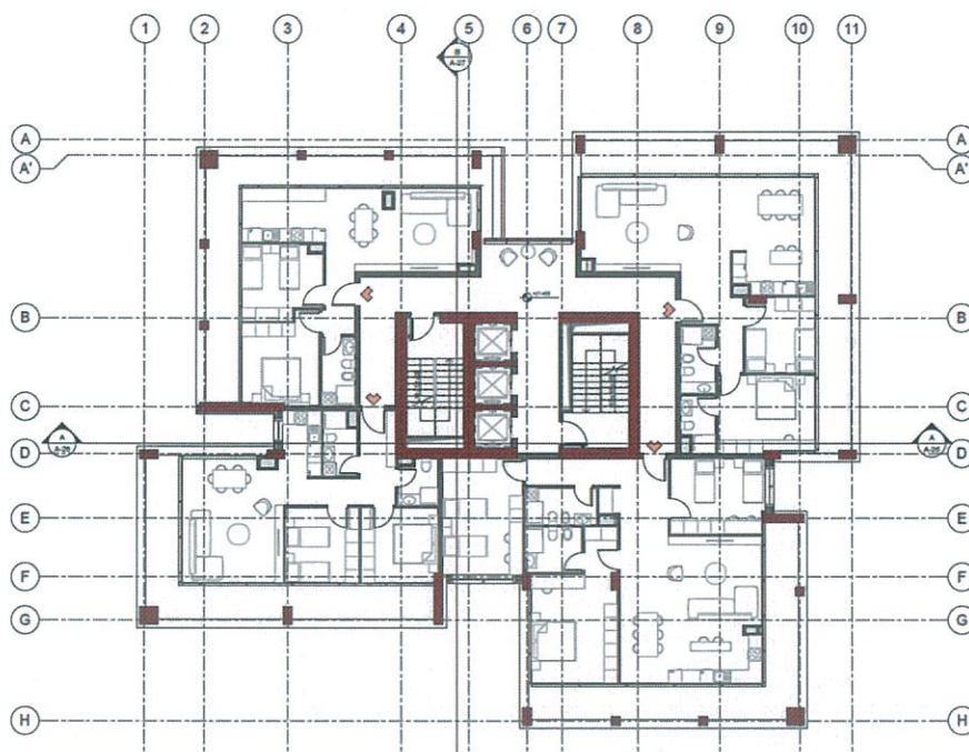
Fig. 10 – Plani i Katit +5 - Banim, Kuota +21.42
