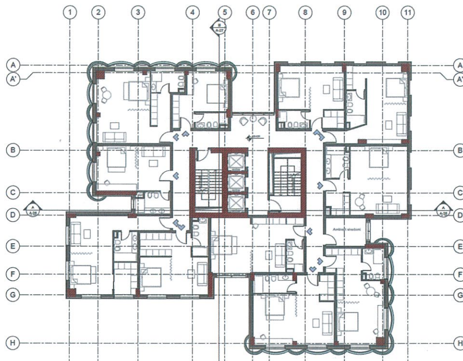
Fig. 12 – Plani i Katit +15 - Hotel, Kuota +55.62
