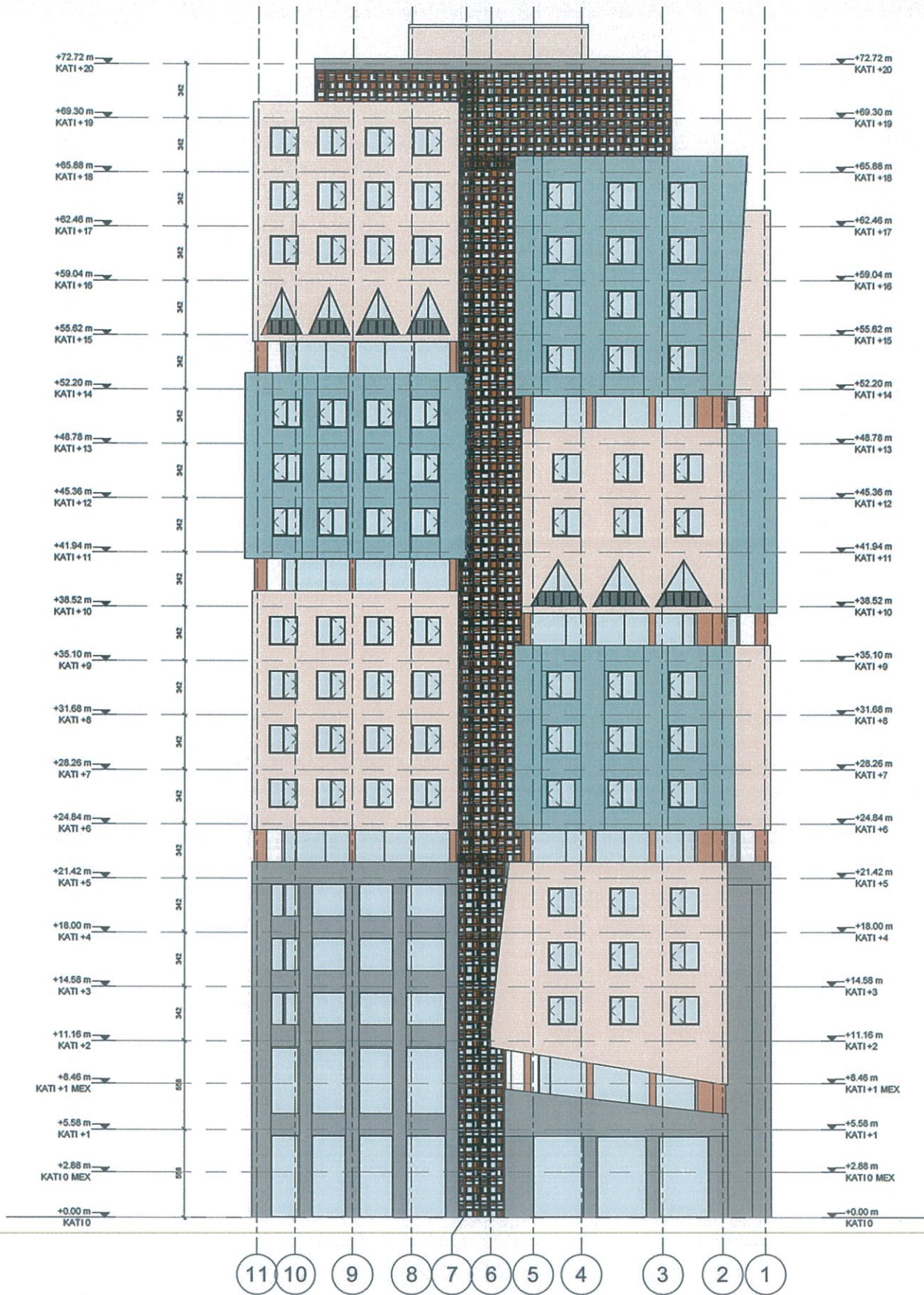
Fig. 18 – Fasada Veriore
