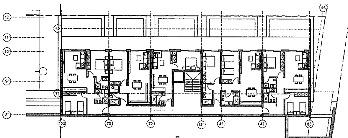
Planimetria e katit të parë
