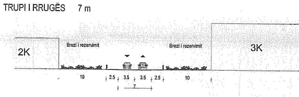
Fig 28. Seksion e rrugës së kategorisë C sipas PPV-së së Bashkisë Durrës
