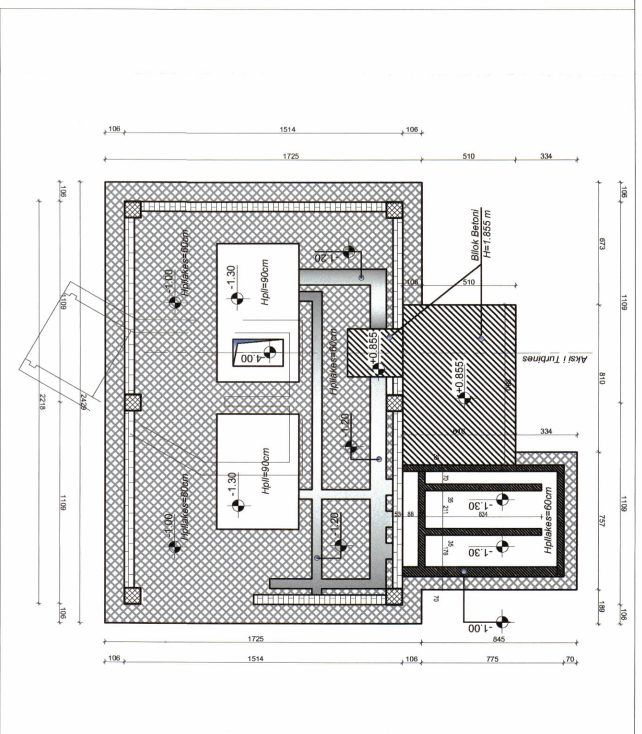
PLANIMETRIA E GODINËS CENTRALIT SHK. 1:200
