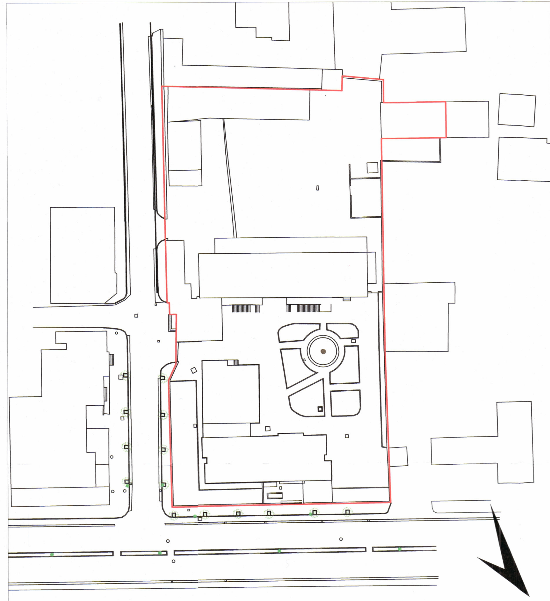
HARTA TOPOGRAFIKE SHK. 1:500
