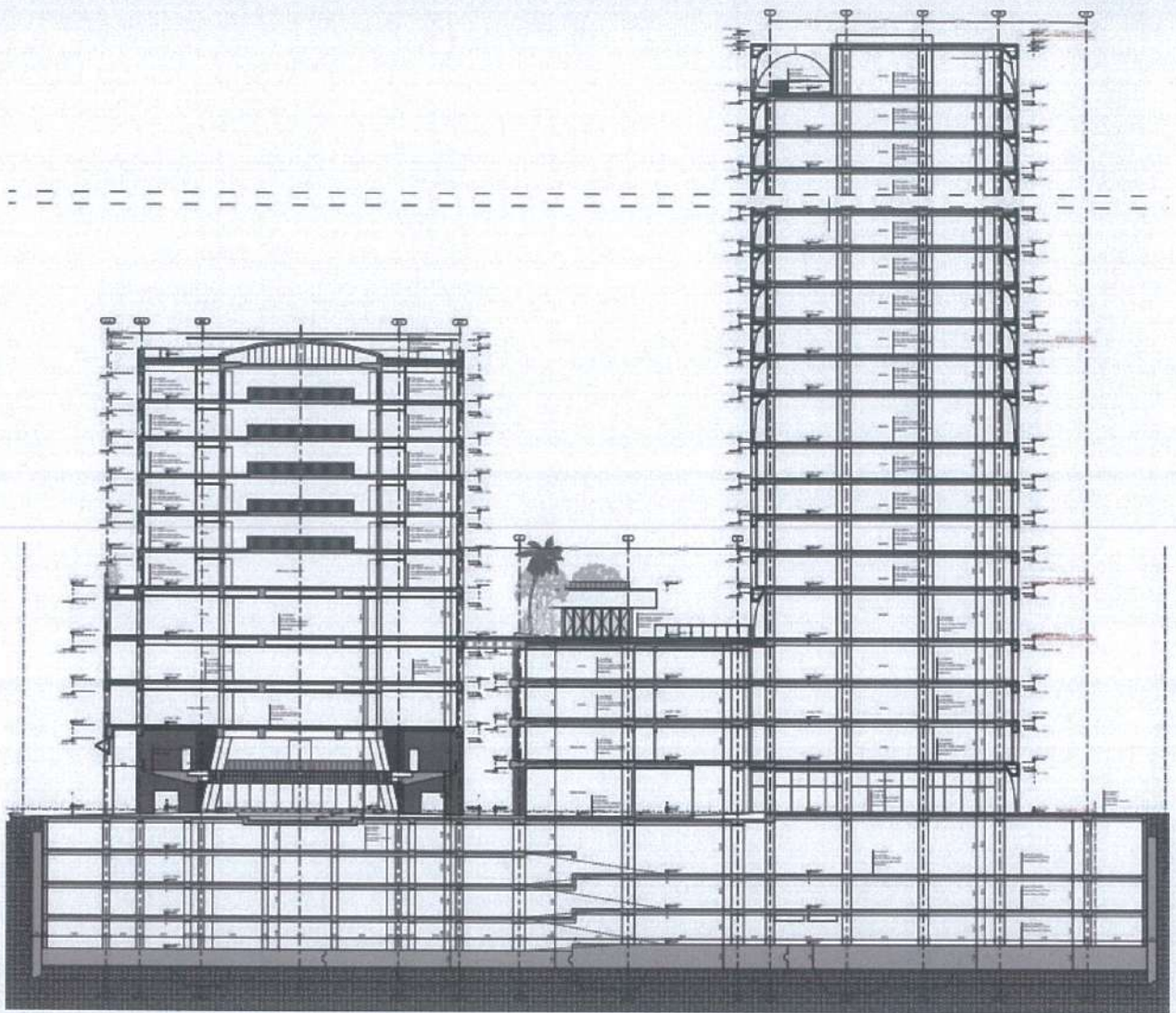
Figure 10 Prerje gjatesore
