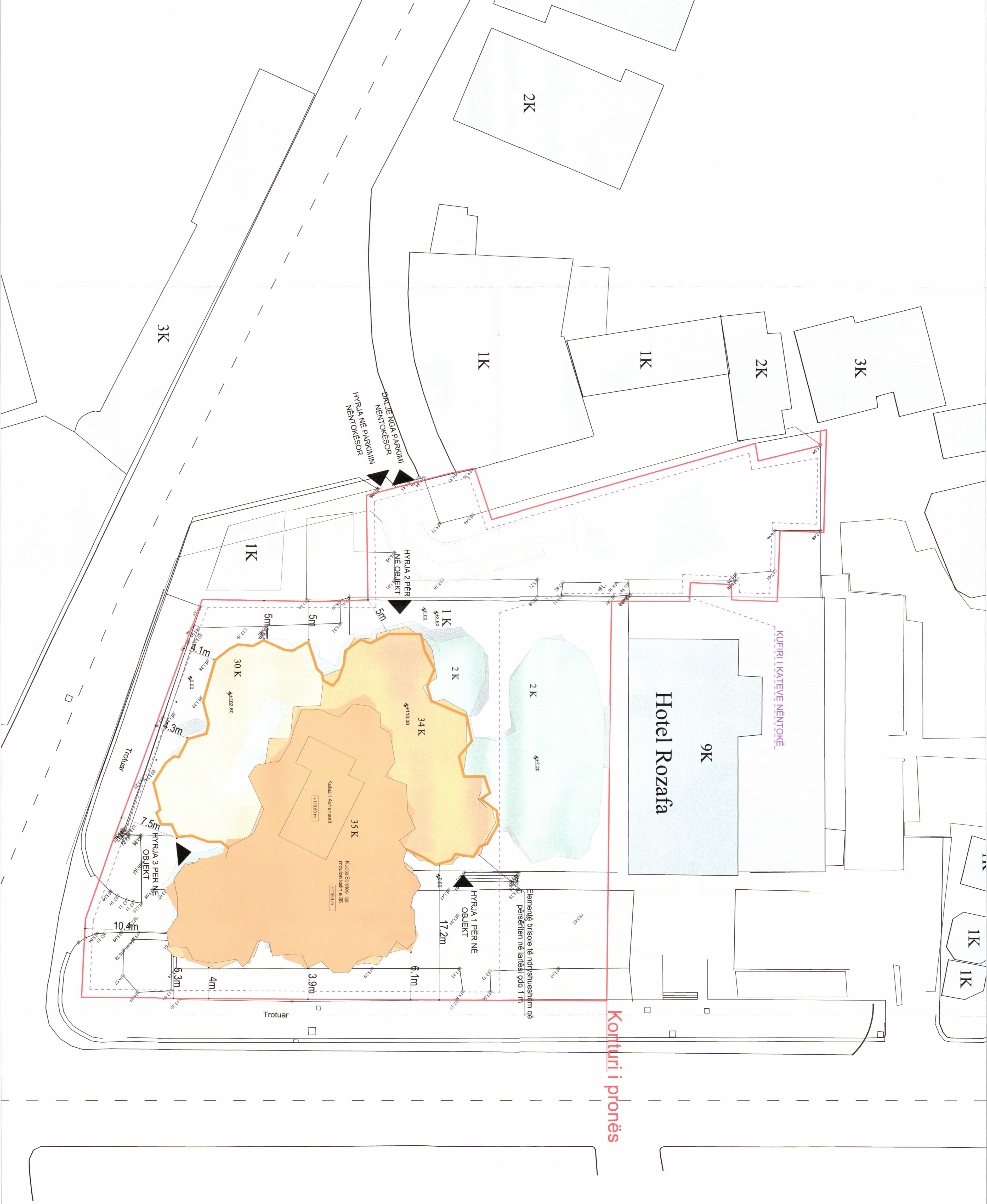
PLANI I VENDOSIES SË STRUKTURËS SHK. 1: 250
