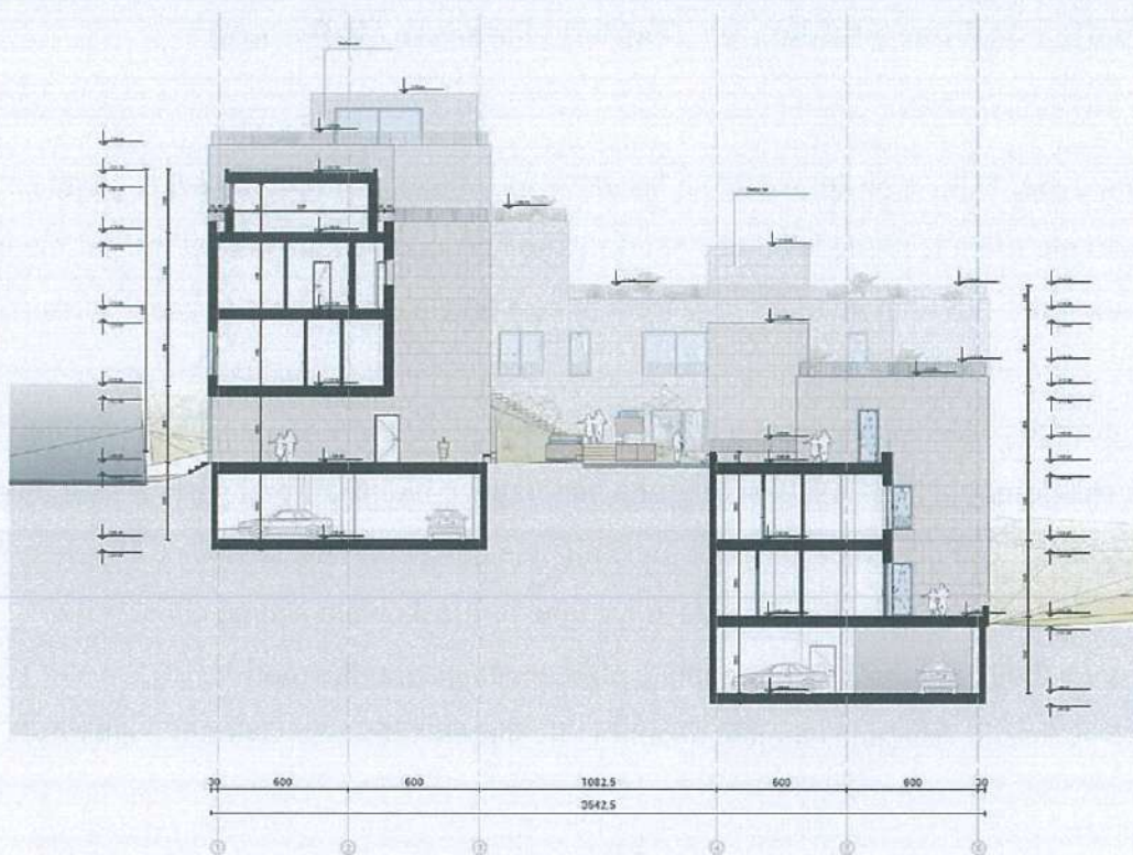
Fig.15 Prerje Tërthore
