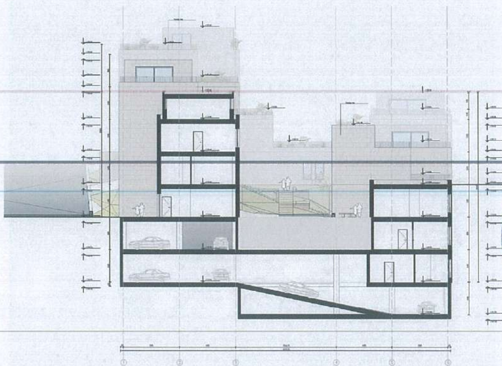
Fig.16 Prerje Tërthore
