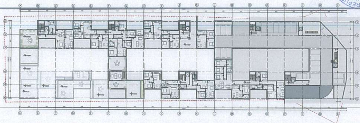
Fig.31. Planimetria e katit në kuotën +115.50.
