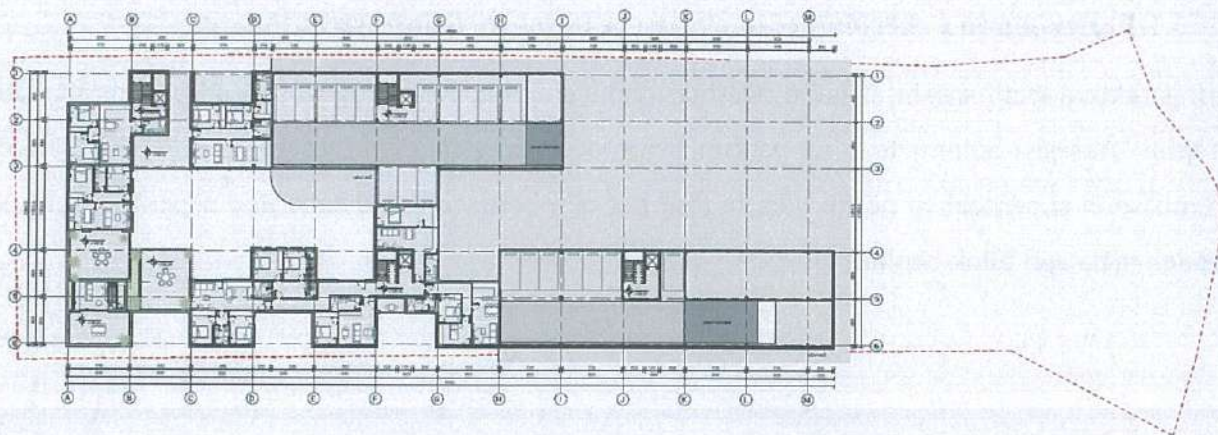
Fig.29. Planimetria e katit në kuotën +108.50.
