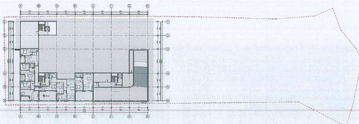
Fig.27. Planimetria e katit në kuotën +101.50.
