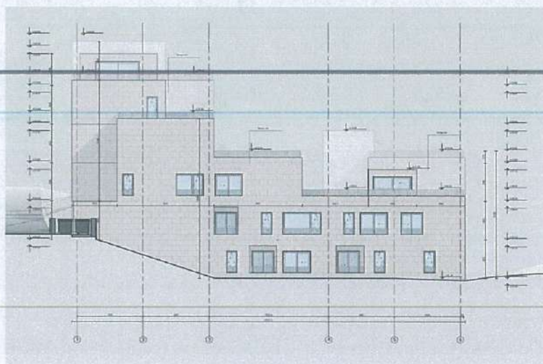
Fig.20 Fasada Jugore
