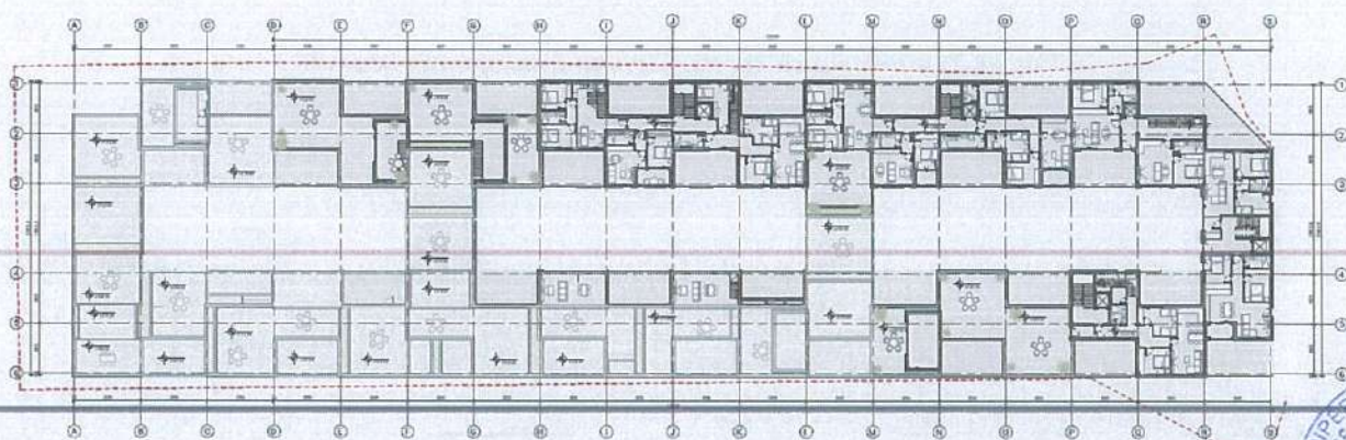
Fig.10 Planimetria në kuotën +122.50
