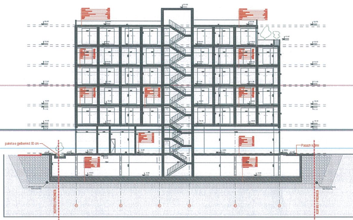
Fig.15 – Prerje e godinës së hotelit
