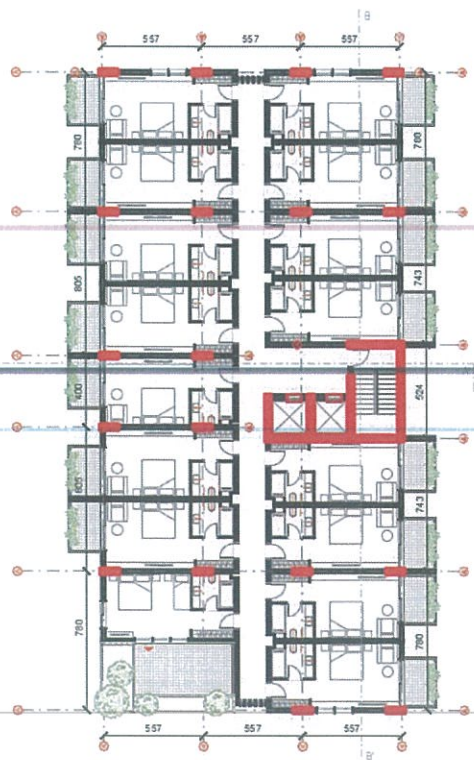
Fig.6 – Planimetri e katit të katërt të objektit të hotelit (+15.00) – 629.1m 2
