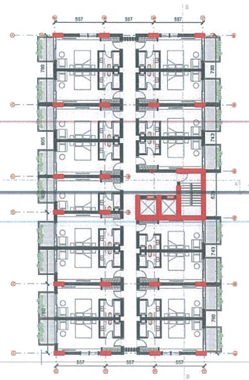
Fig.4 – Planimetri e katit të dytë të objektit të hotelit (+8.00) – 700.8m 2
