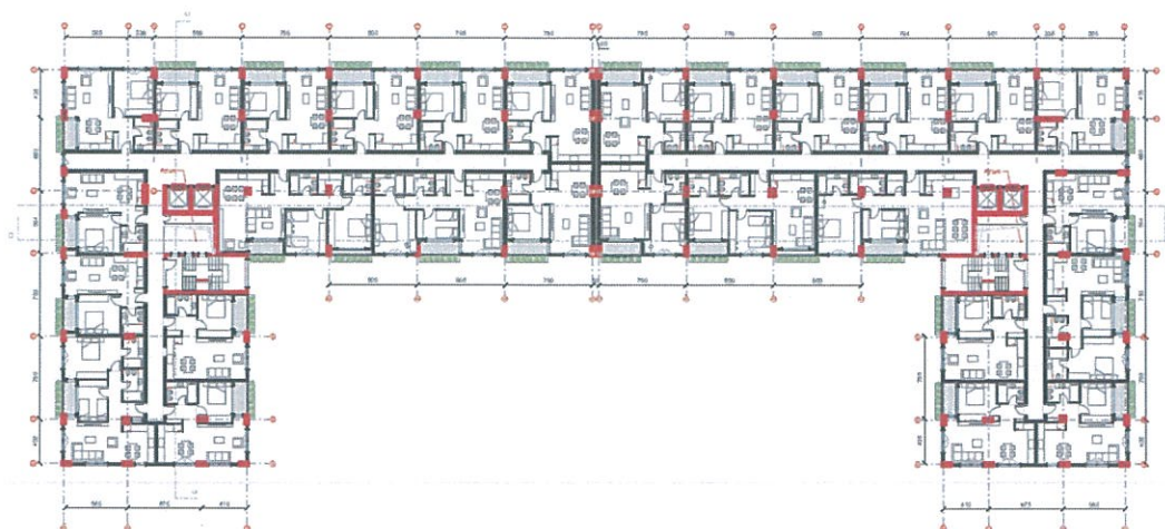
Fig.9 – Planimetri e katit të dytë të objektit të apartamenteve (+3.23) – 2295m 2
