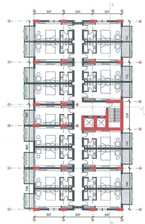
Fig.5 – Planimetri e katit të tretë të objektit të hotelit (+11.50) – 688.2m 2
