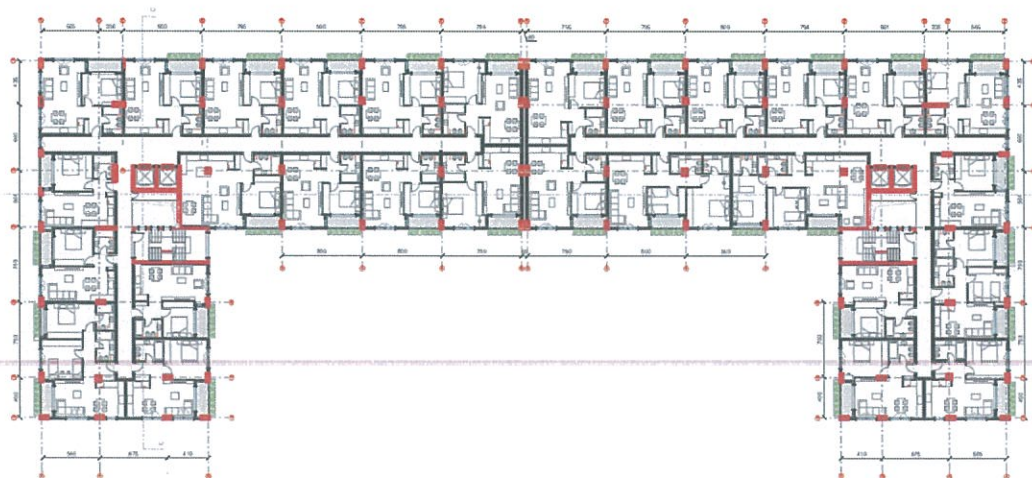
Fig.10 – Planimetri e katit të tretë të objektit të apartamenteve (+6.46) – 2295m 2
