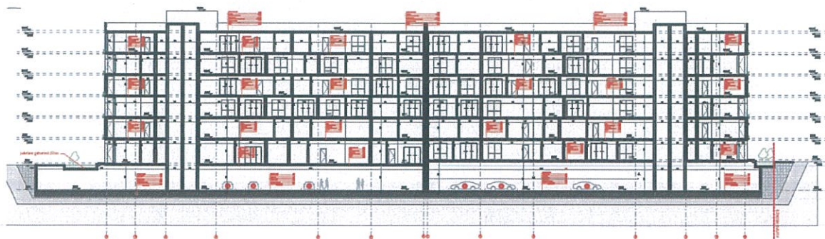
Fig.14 – Prerje e godinës së apartamenteve
