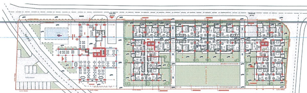
Fig.2 – Plansistemi i katit përdhe
