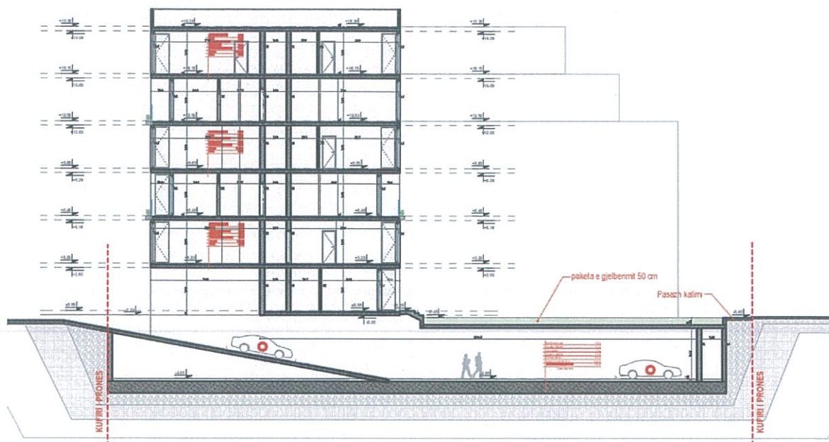
Fig.16 – Prerje e godinës së apartamenteve përgjatë rampës së parkimit
