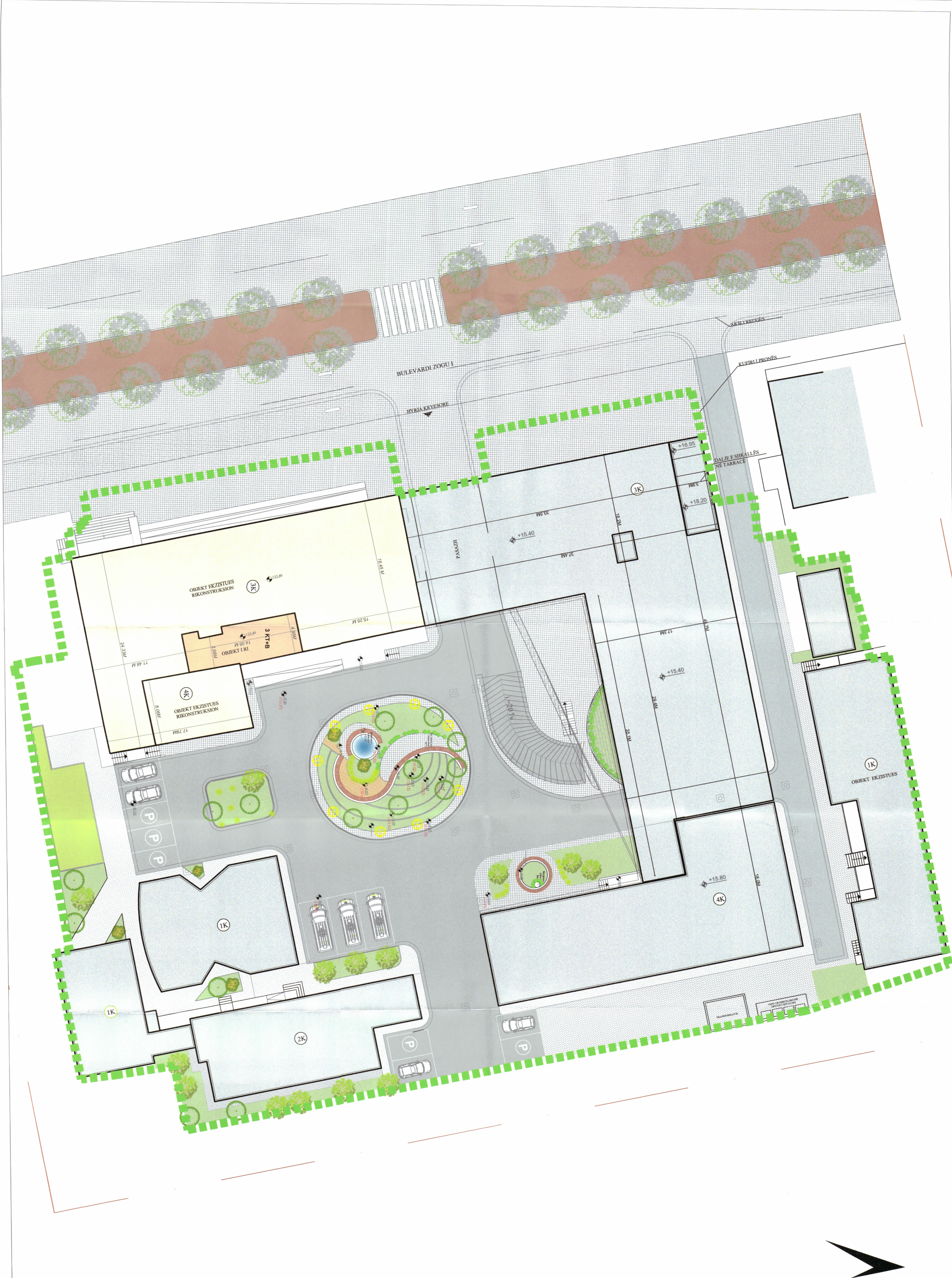
PLANI I VENDOSJES SË STRUKTURËS SHK. 1:300
