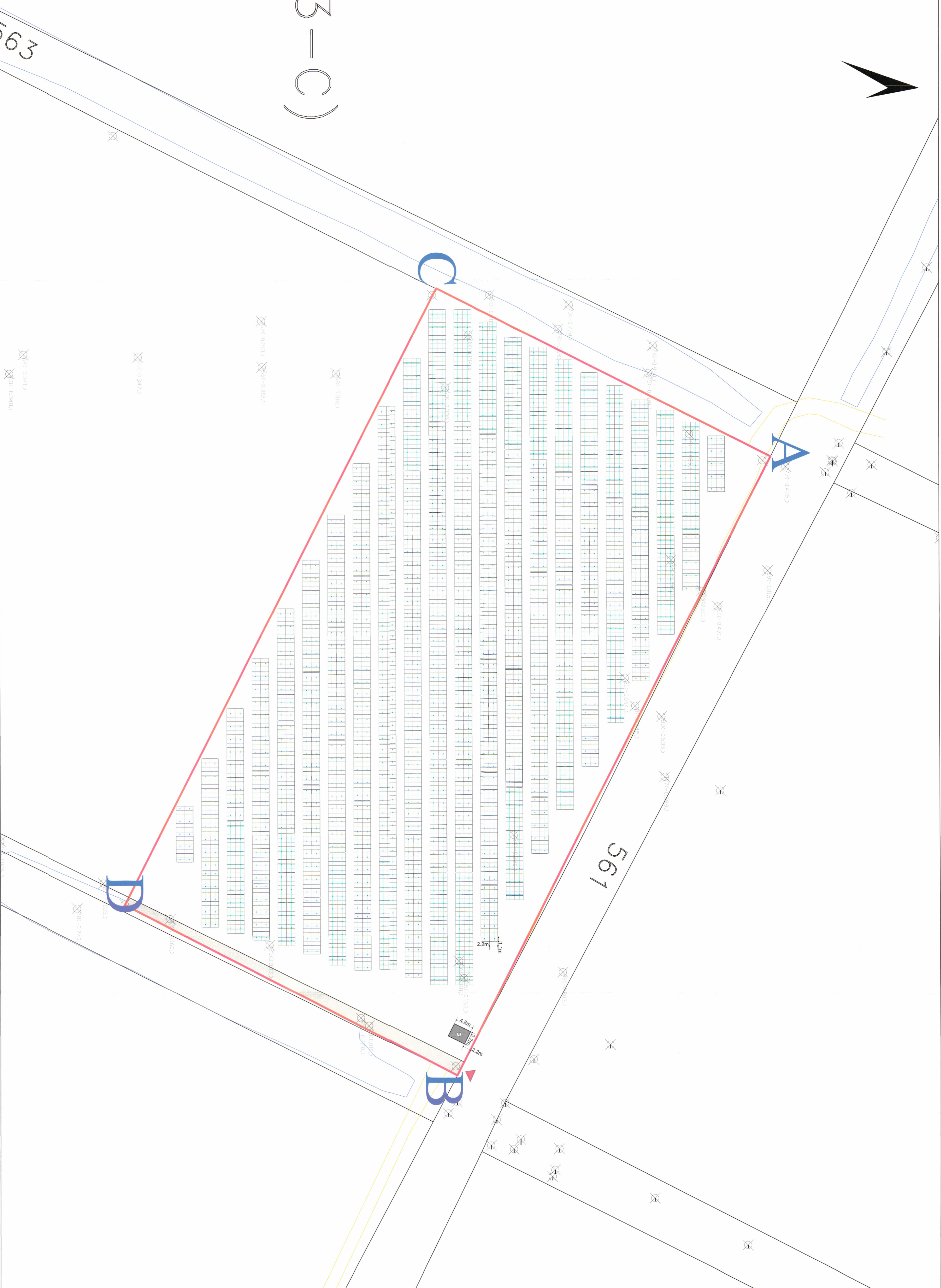
PLANI I VENDOSIES SË IMPIANTIT FOTOVOLTAIK SHK. 1: 500
