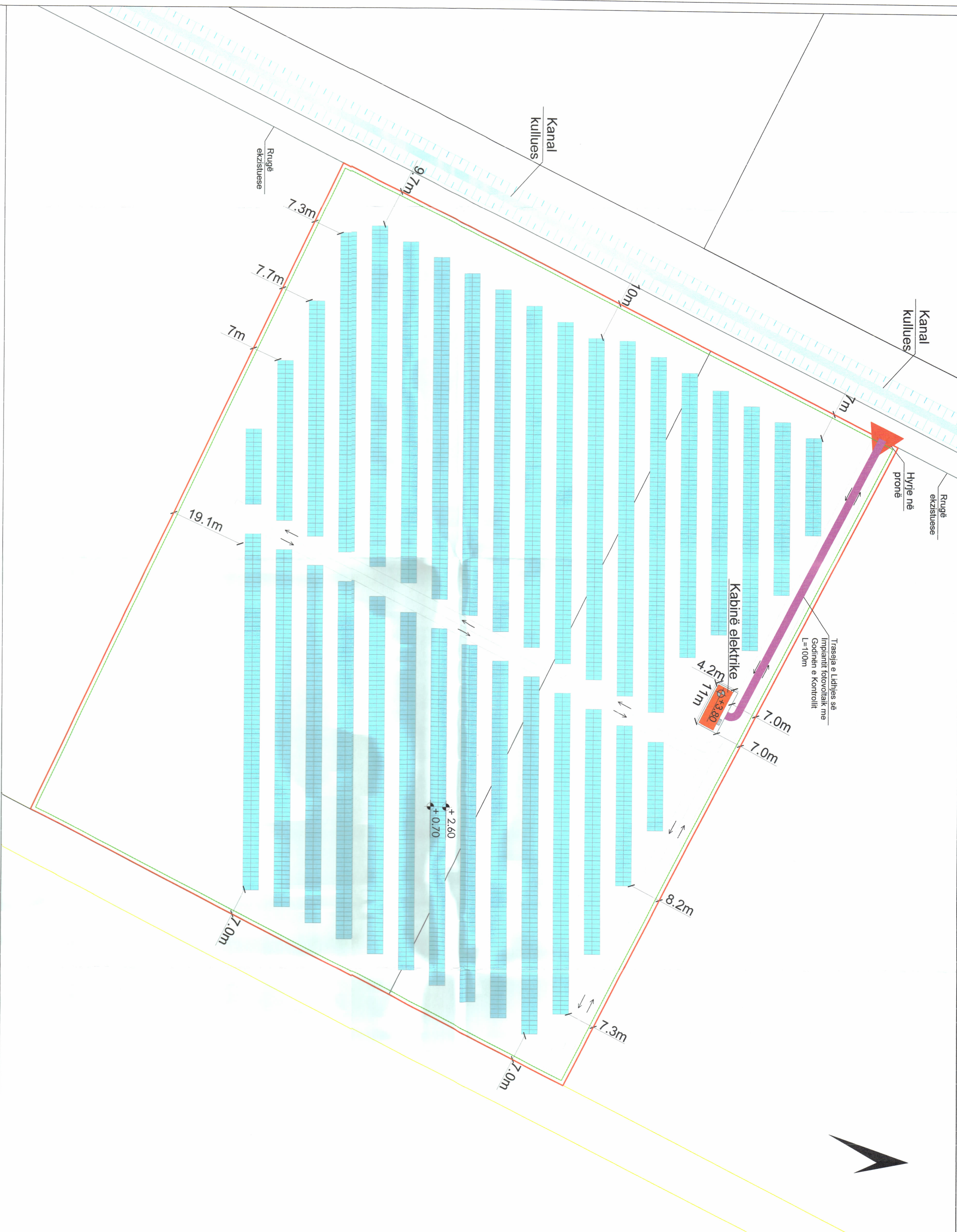
PLANI I VENDOSIES SË IMPIANTIT FOTOVOLTAIK SHK. 1: 500
