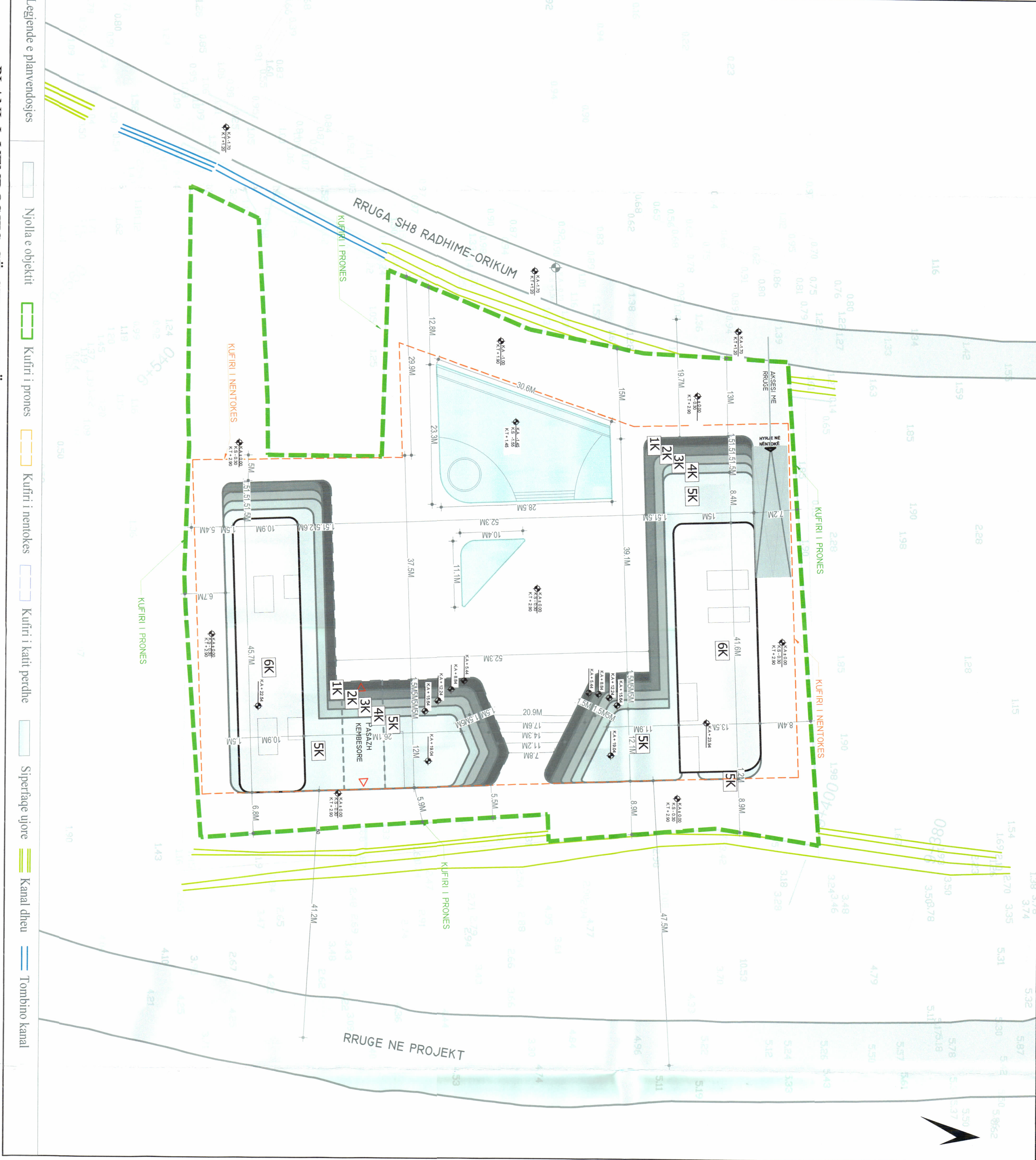
PLANI I VENDOSIES SË STRUKTURËS SHK. 1:500
