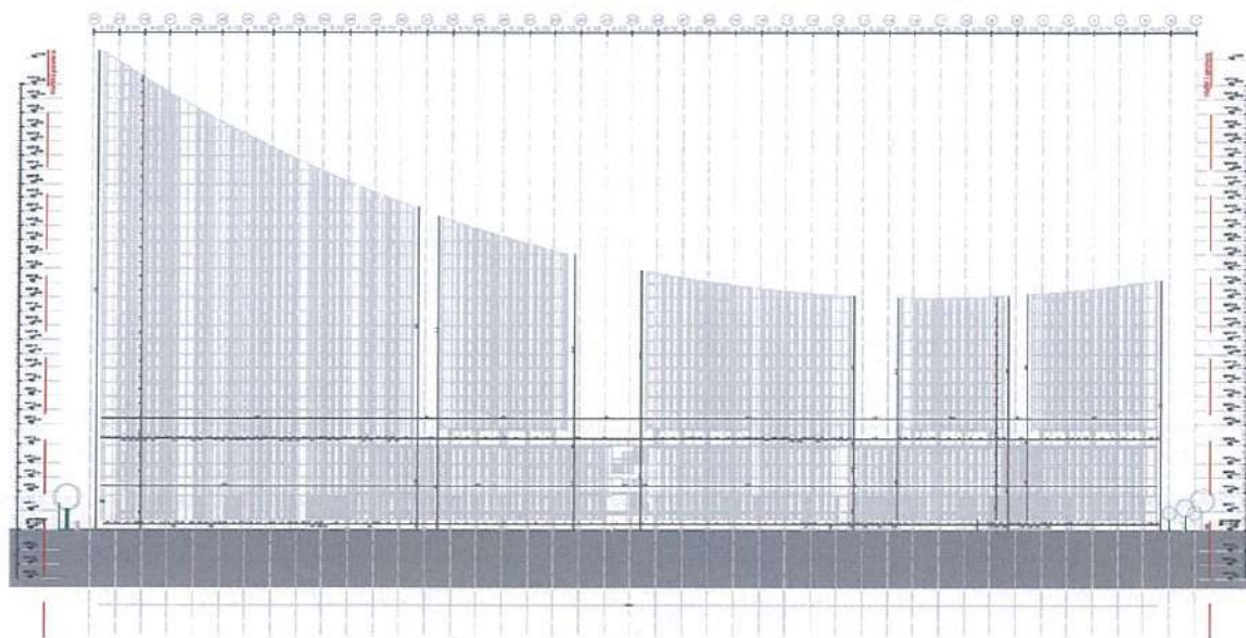
Figura 17 Fasada Veriore
