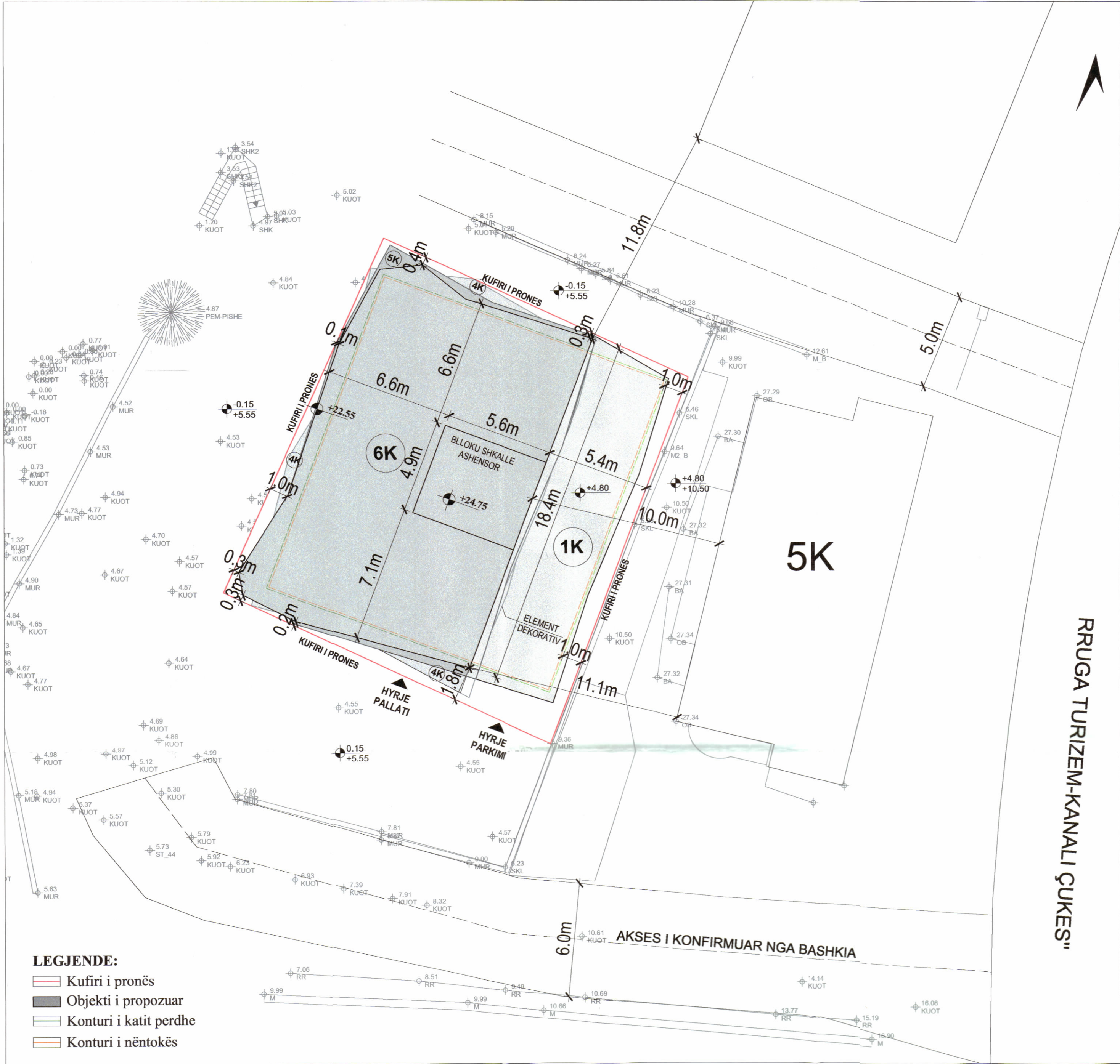
PLANI I VENDOSJES SË STRUKTURËS SHK. 1:150
