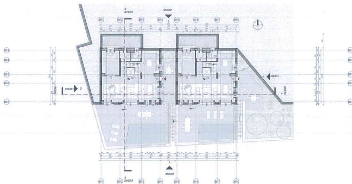
Fig. 18 – S-7 – Plani i katit përdhe
