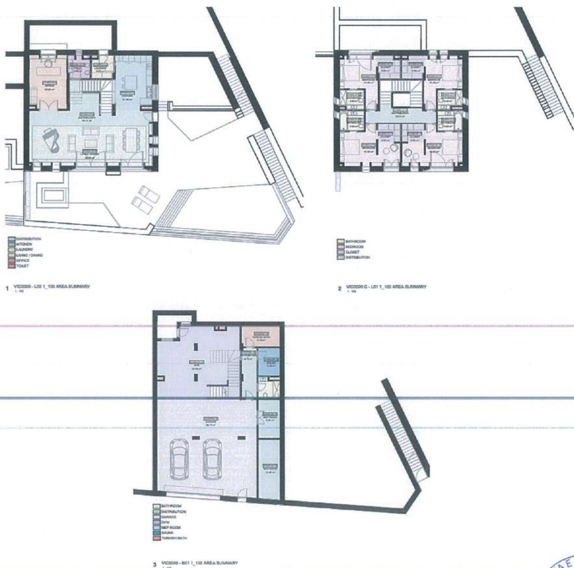
Fig. 17 – Planet e vilës tip C
