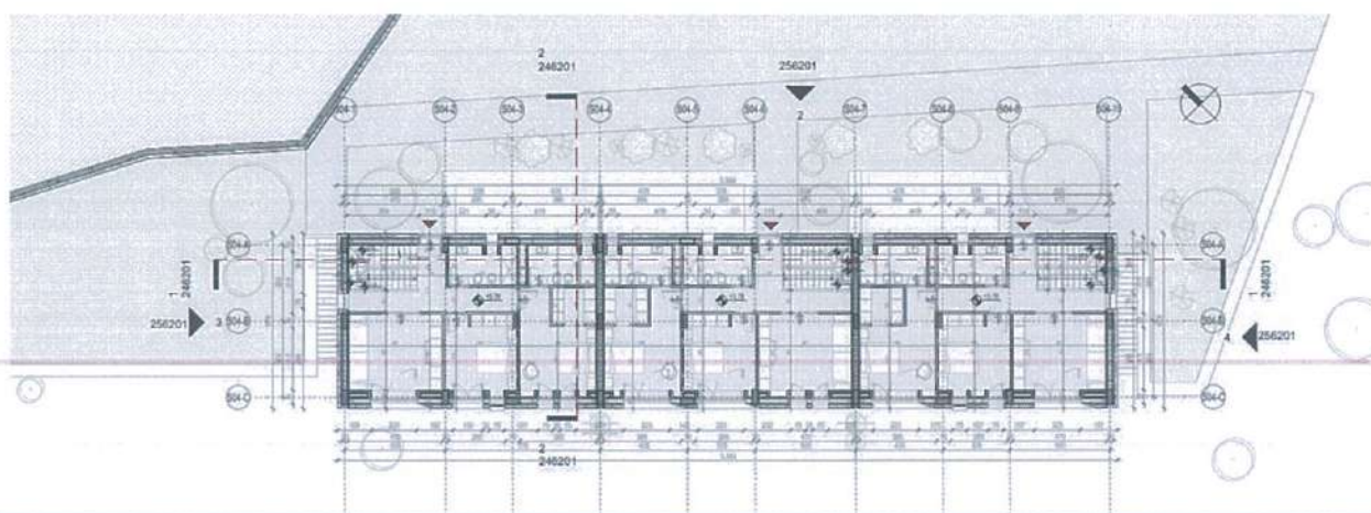
Fig. 15 – S-4 – Plani i katit të parë
