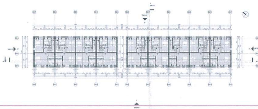
Fig. 11 – S-2 – Plani i katit të parë
