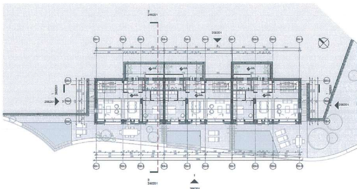
Fig. 14 – S-4 – Plani i katit përdhe
