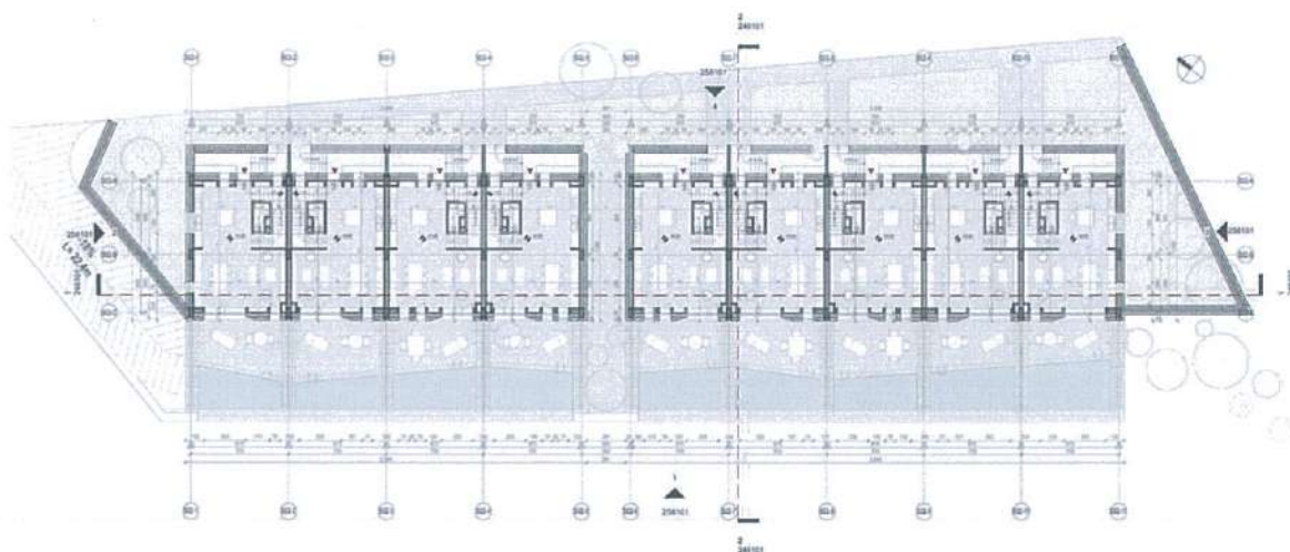
Fig. 10 – S-2 – Plani i katit përdhe
