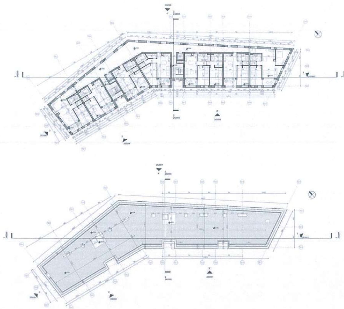
Fig. 21 T-2 Plani i katit +3 dhe mbulesës
