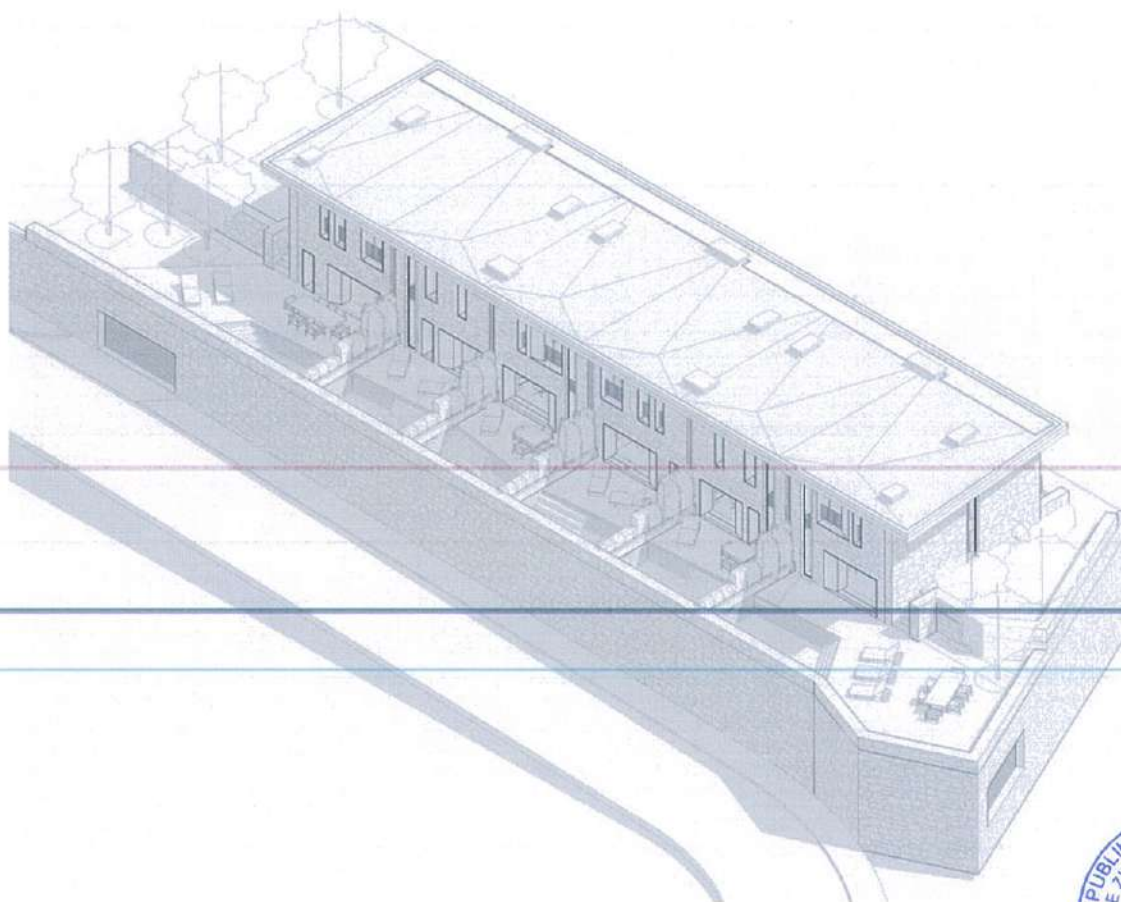
Fig. 25 – Volumetri – S-8, Vilë Tip A
