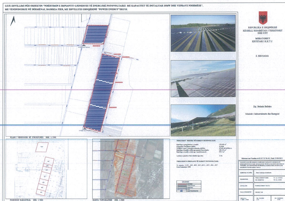
Figura 7. Planvendosja e strukturës që propozohet
