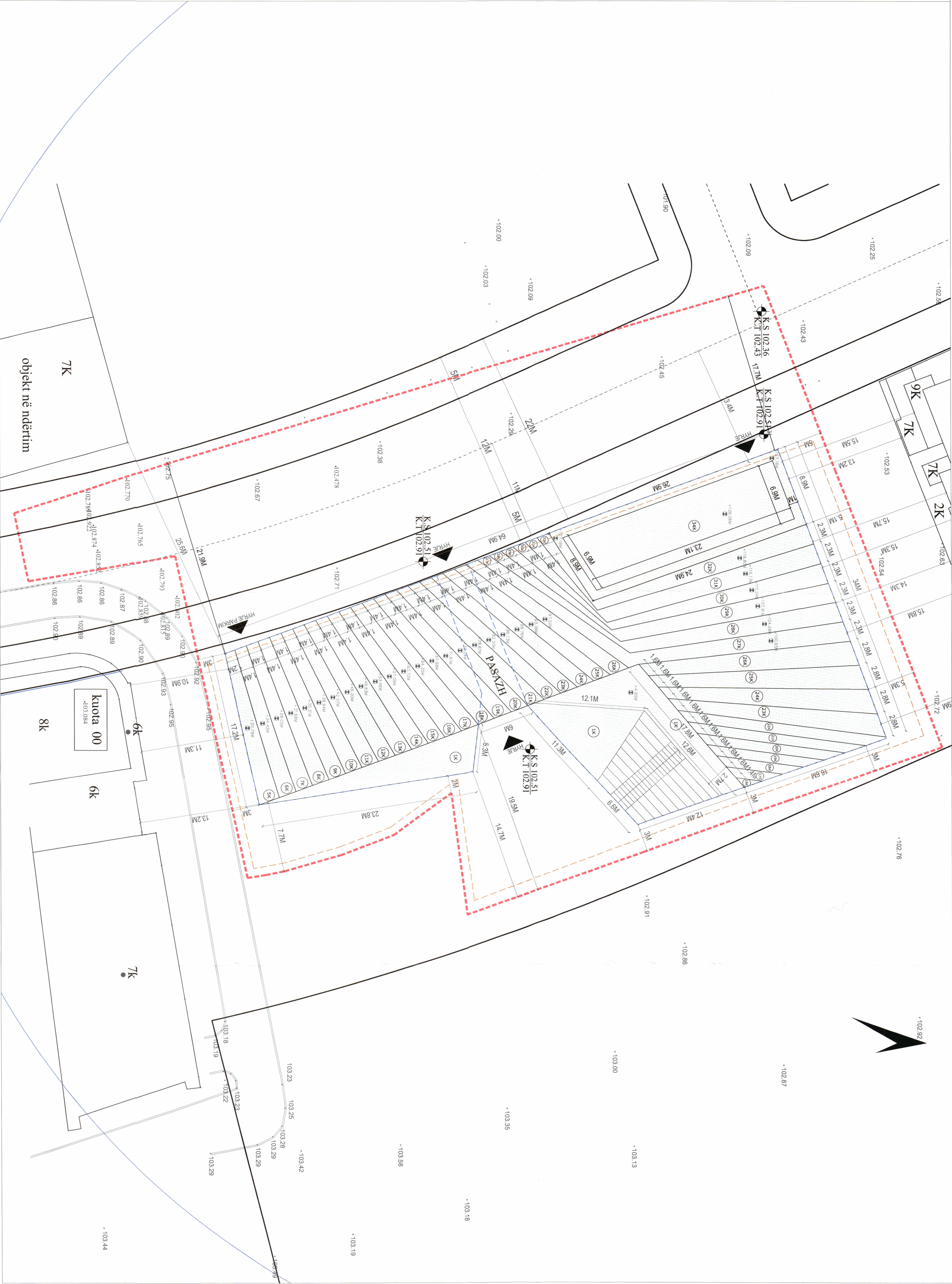
PLAN I VENDOSJES SË STRUKTURËS SHK. 1: 200
