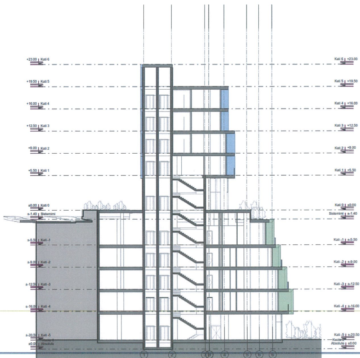
Fig. 12. Prerje
