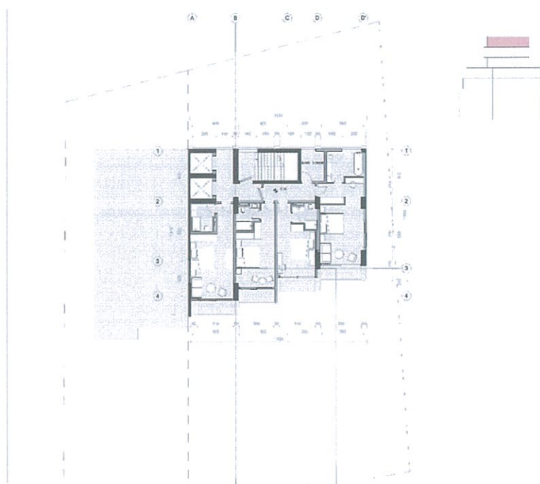
Fig. 10. Plani i katit tip per katet mbi nivelin \pm 0.00
