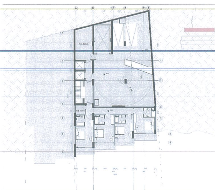
Fig. 11. Plani i katit tip për katet nën nivelin \pm 0.00
