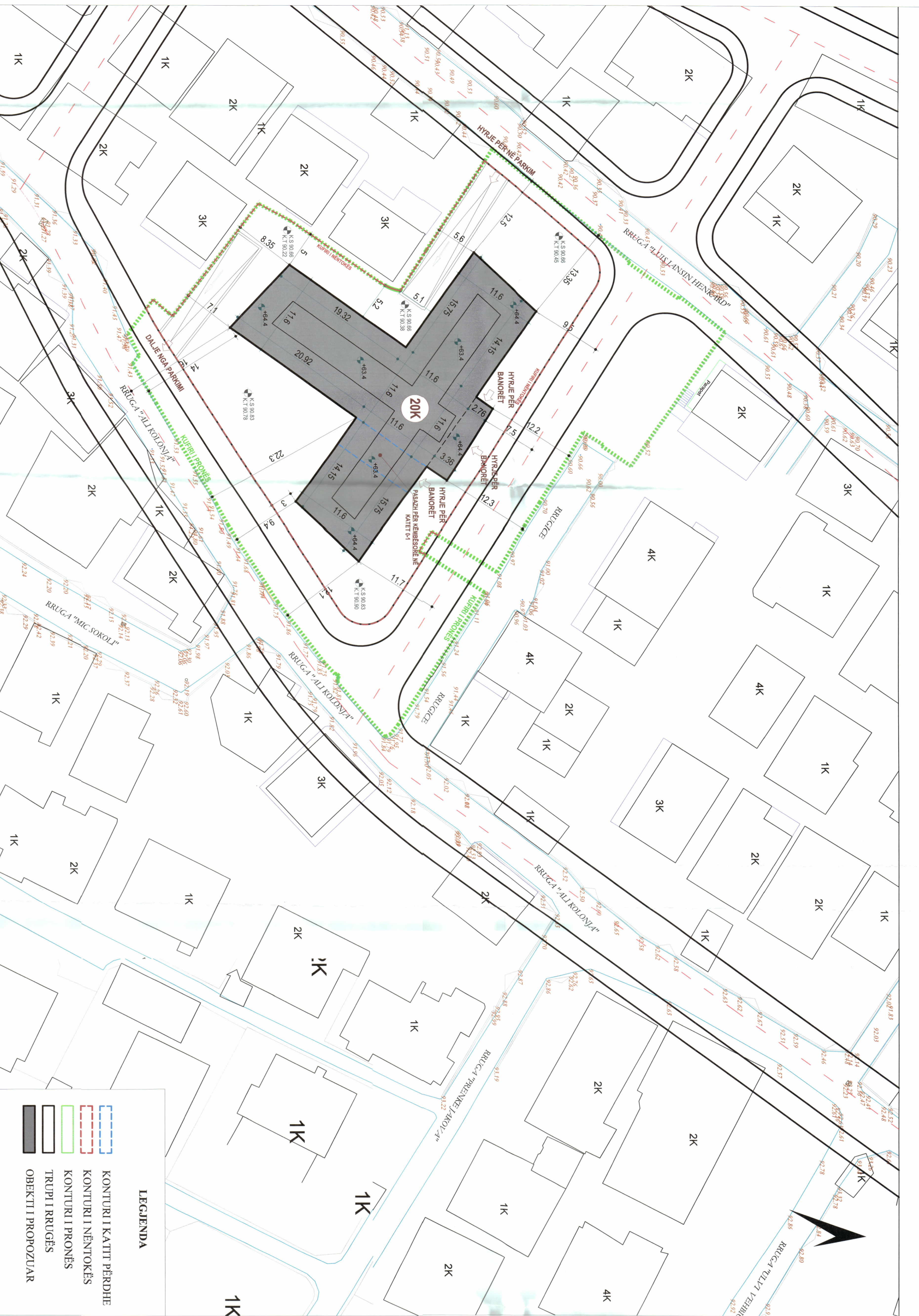
PLANI I VENDOSIES SË STRUKTURËS SHK. 1: 250
