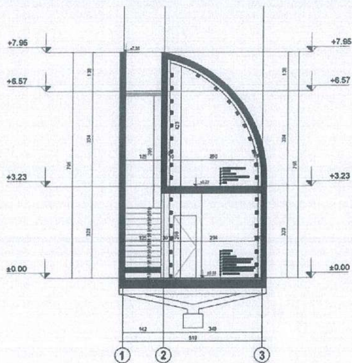
Fig.12. Prerje tërthore-Kabina akomoduese
