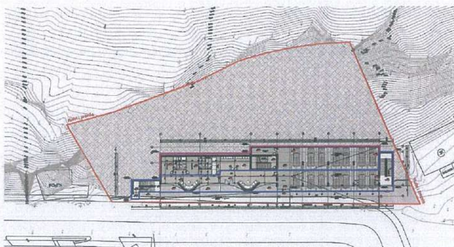
Fig.2 Planimetria në kuotën 0.00, sipërfaqe 661m 2 nga të cilat 345 m 2 mbi tokë dhe 316 m 2 nëntokë
