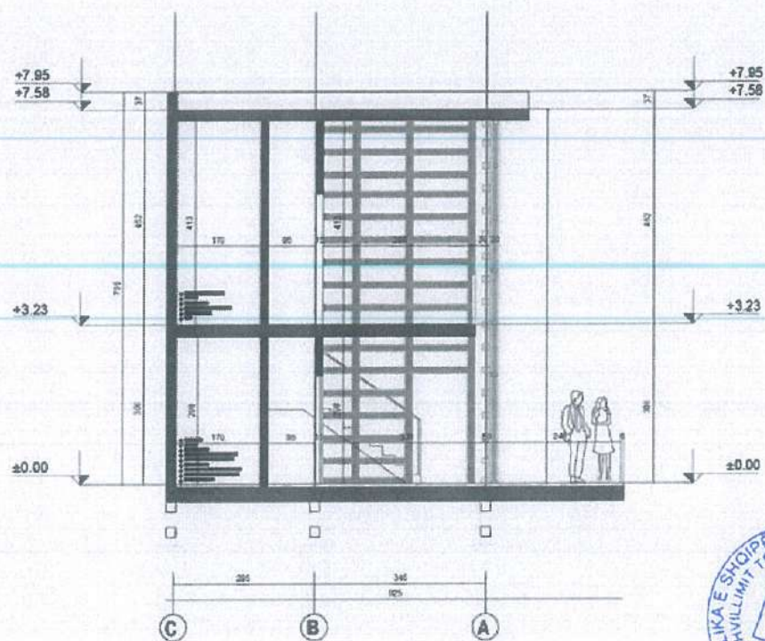
Fig.13. Prerje gjatësore-Kabina akomoduese
