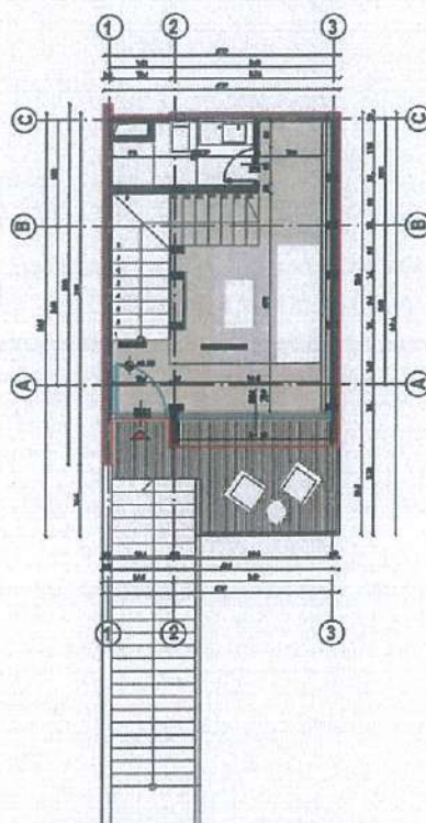
Fig.4 Kabina/ Planimetria e katit përdhe , sipërfaqe 37.3m 2
