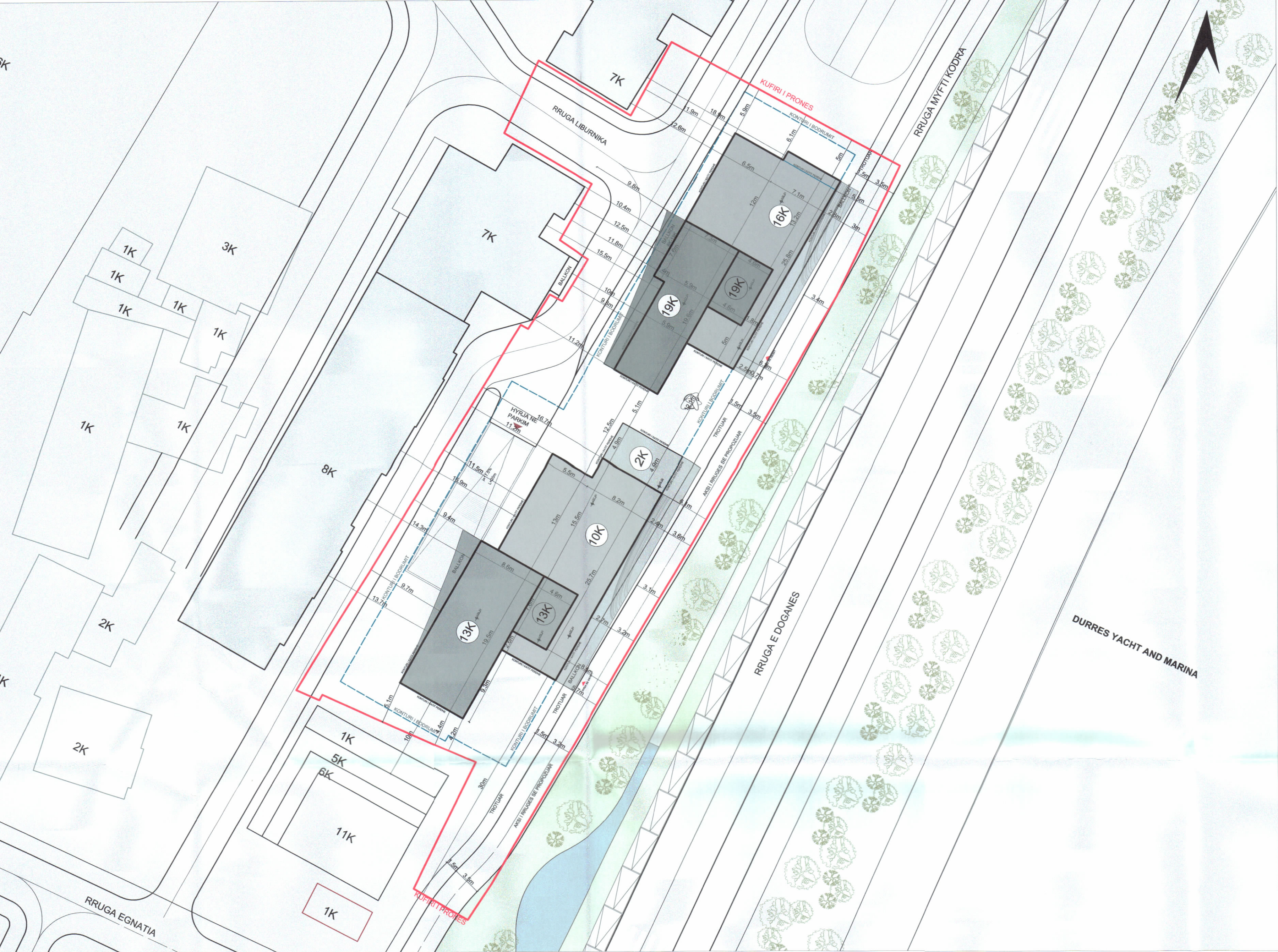
PLANI I VENDOSJES SË STRUKTURËS SHK. 1:350
