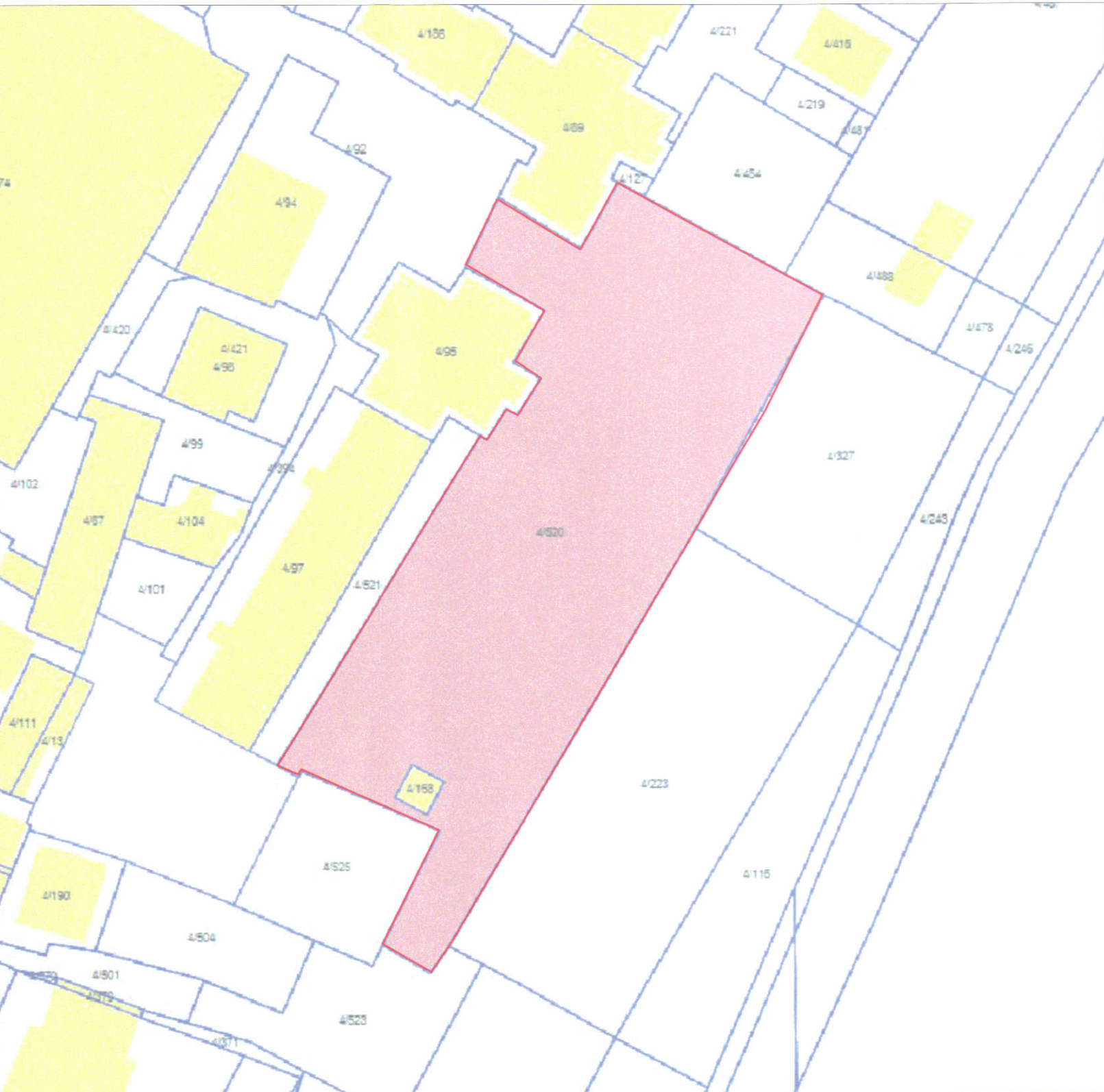
POZICIONI KADASTRAL SHK. 1:750
