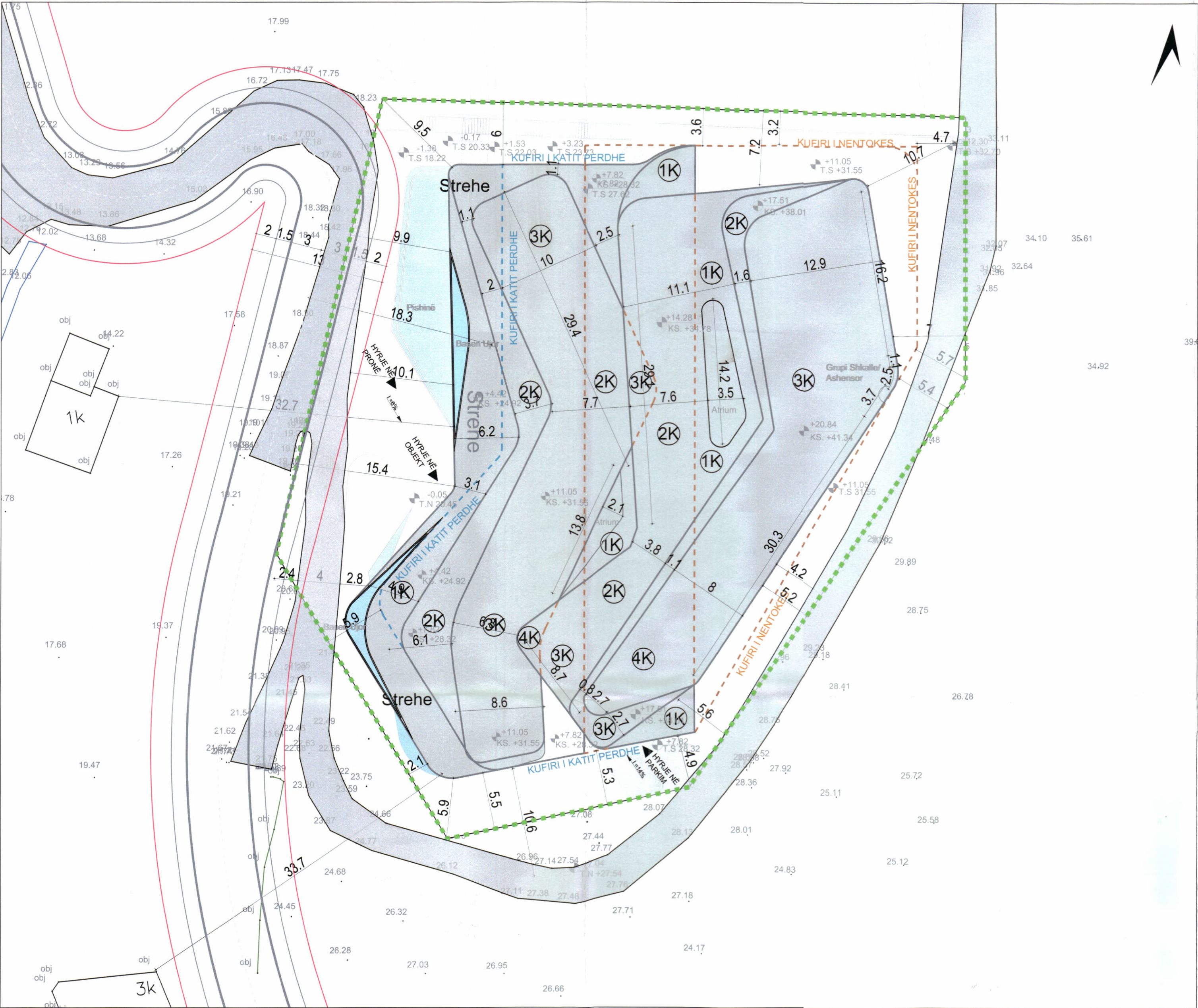
PLANI I VENDOSJES SË STRUKTURËS SHK. 1:300
